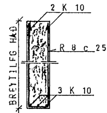
SNID A-A 1:20
