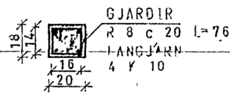
SÚLA S.12 1:20
