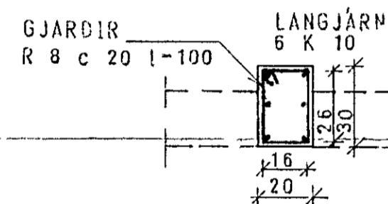
SÚLA S.11 1:20
