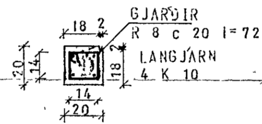
SÚLA S.13 1:20
