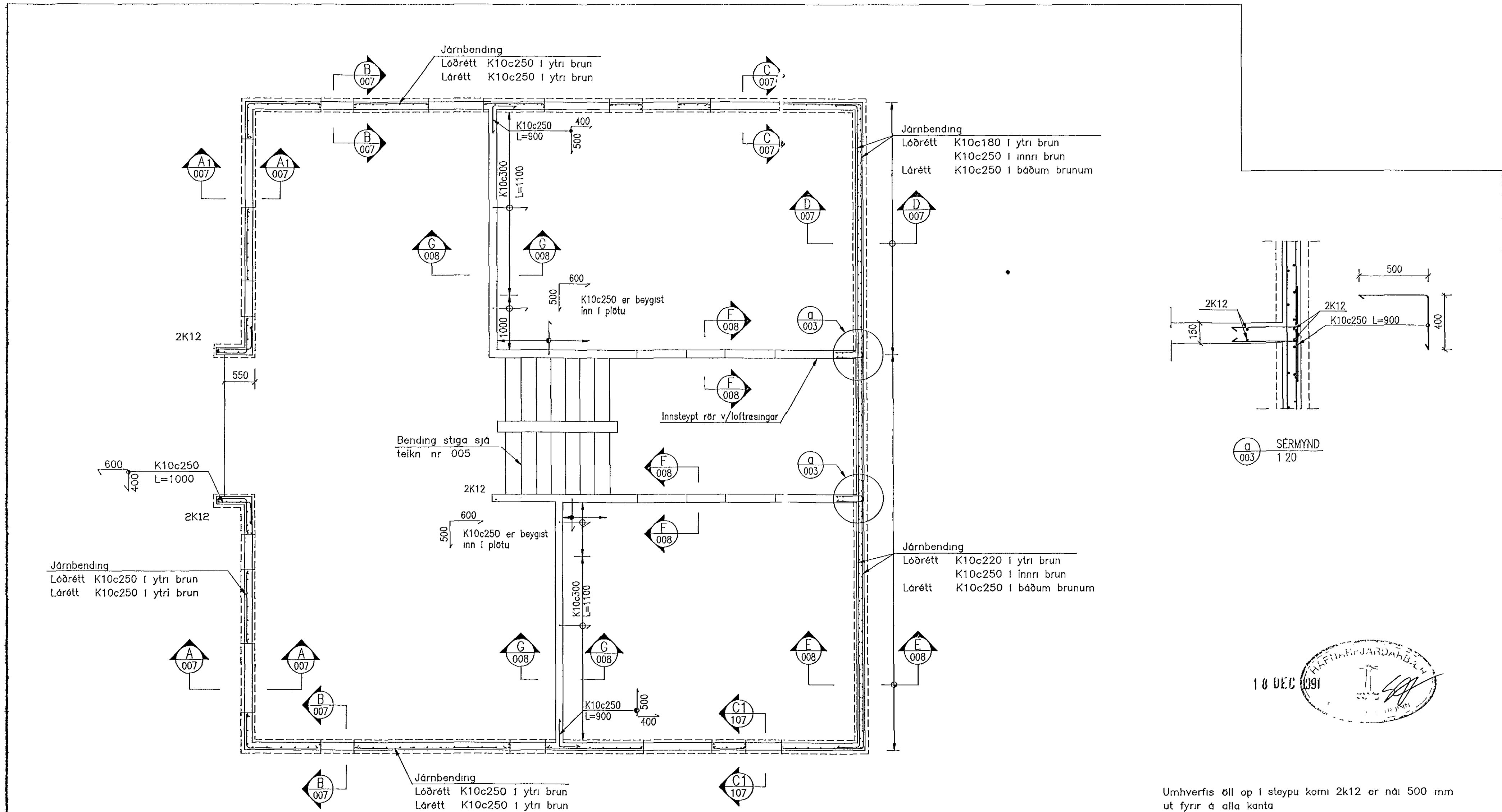
GRUNNMYND 1.50
