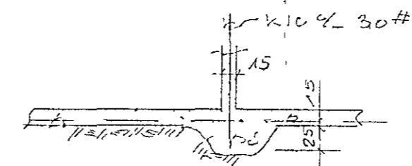
SNID I STIGAVEGG A-A 1:50
