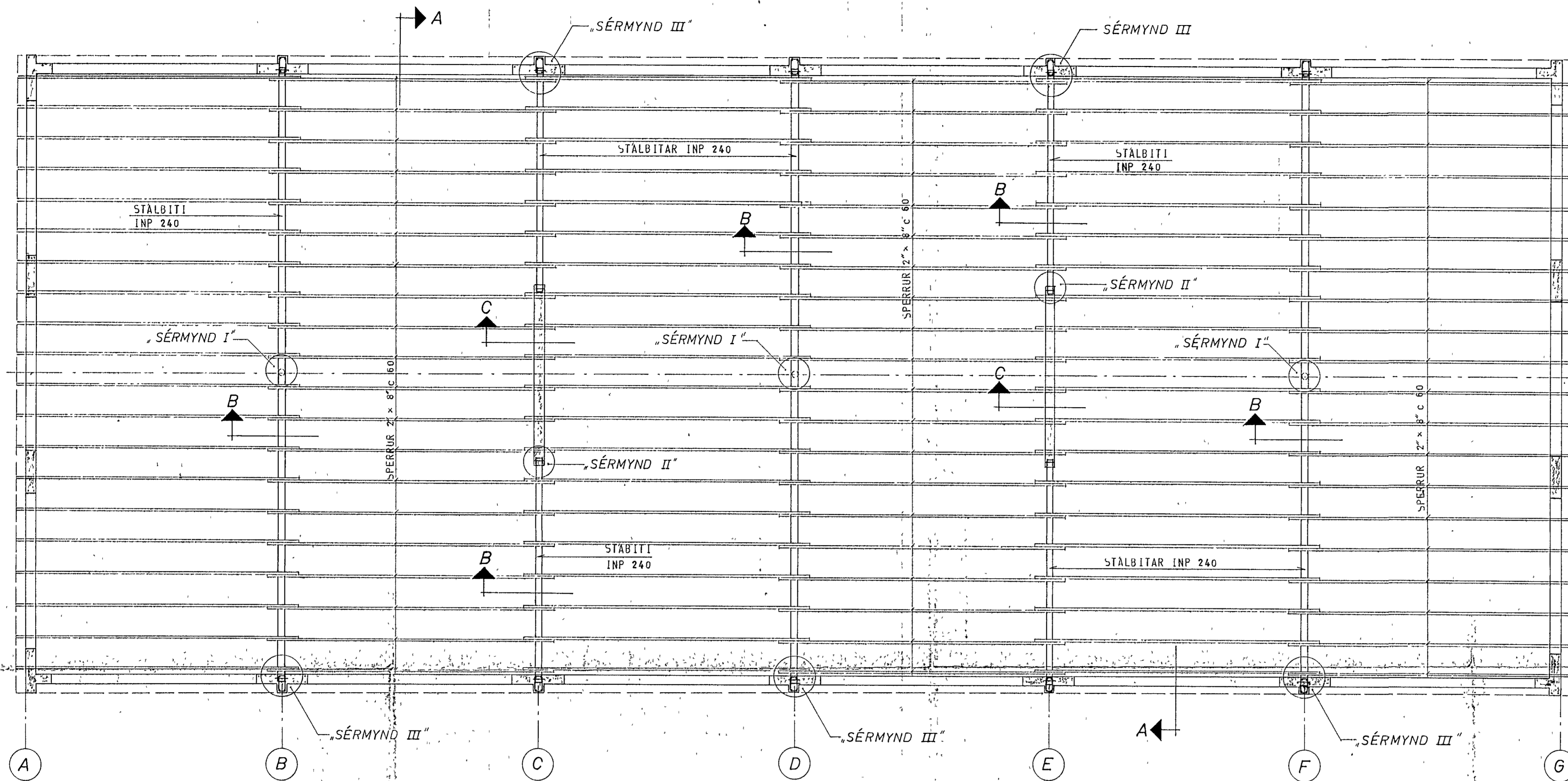
GRUNNMYND ÞAKS 1:50
