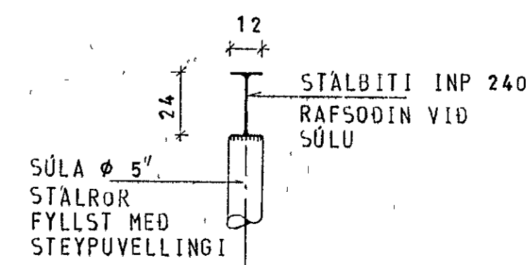
SÉRMYND I 1:20
