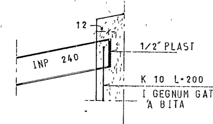
SÉRMYND II 1:20
