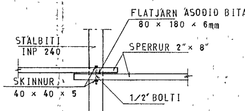
SNID B, 1:20
