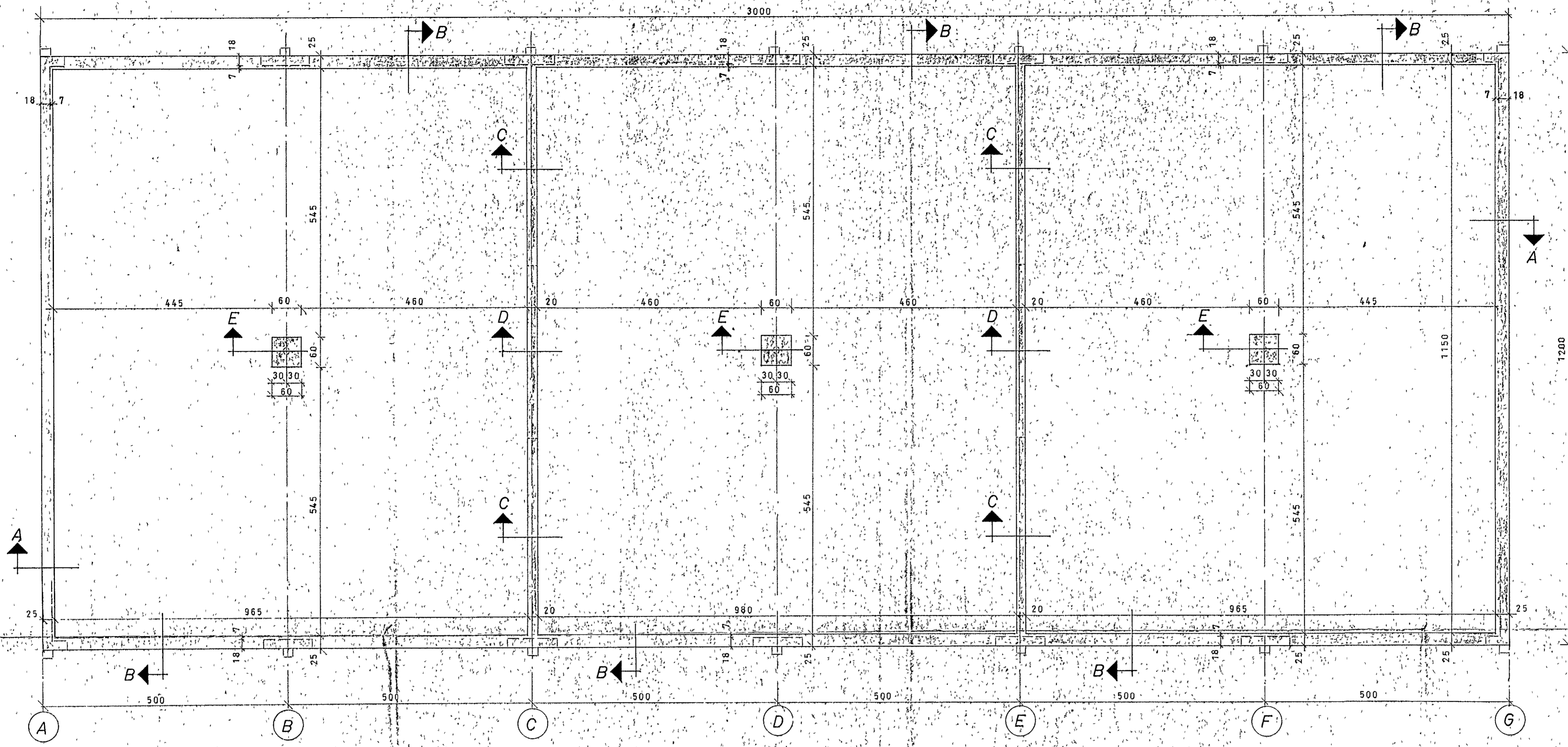
GRUNNMYND - UNDIRSTÖÐUR 1:50
