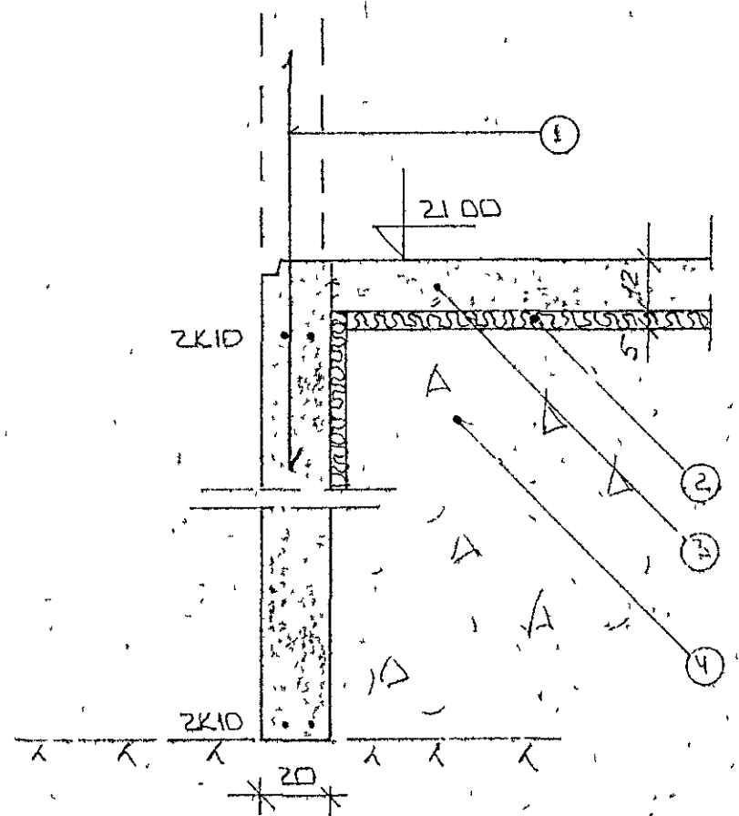
SNID 1 Í UTVEGGI 1:20
