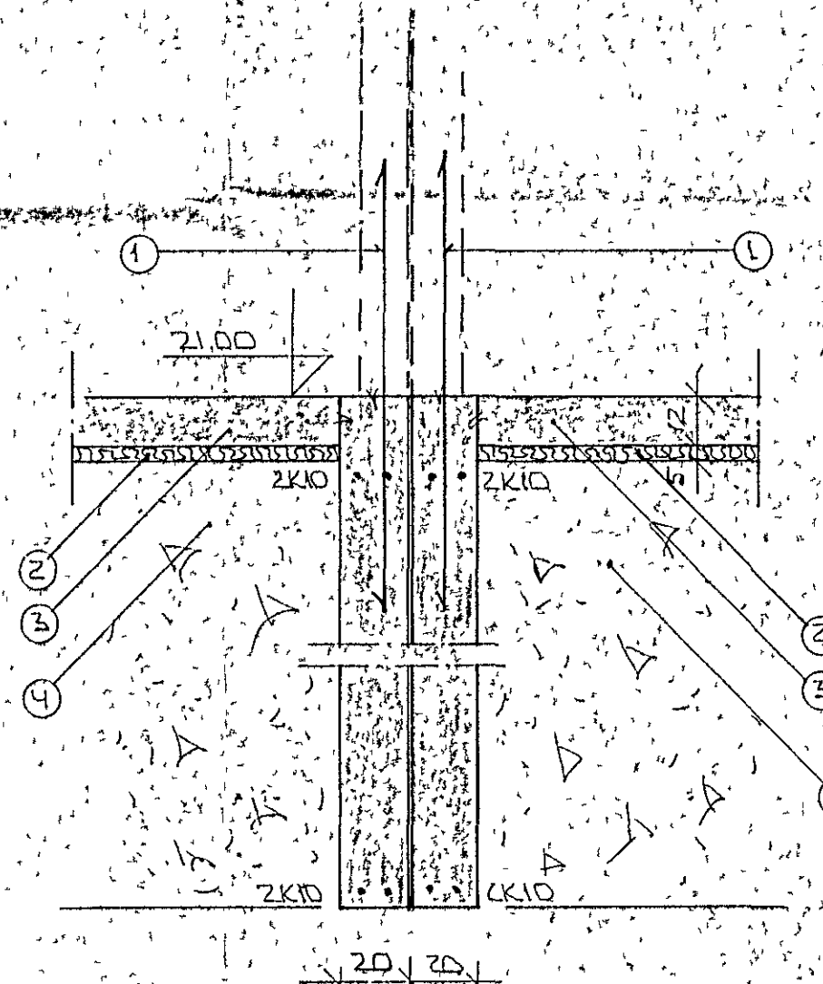
SNID 4 Í VEGGI M/IBUÐA 1:20
