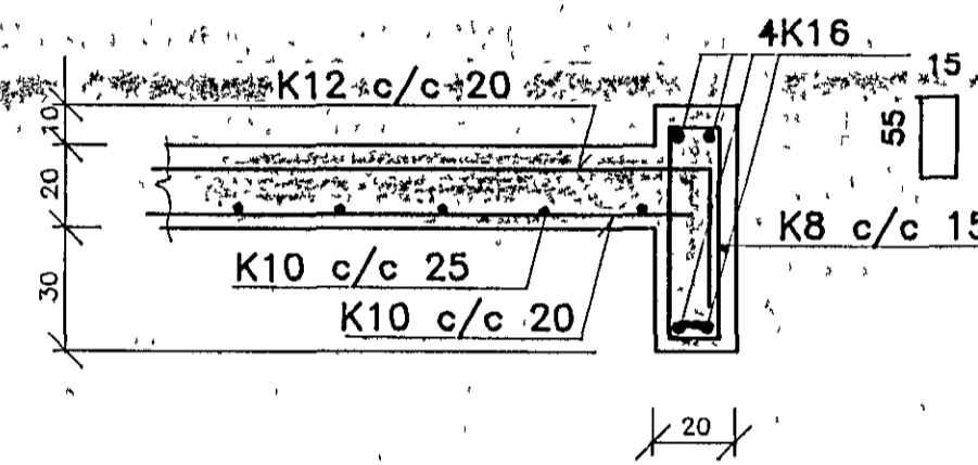
SNID D-D 1:20
