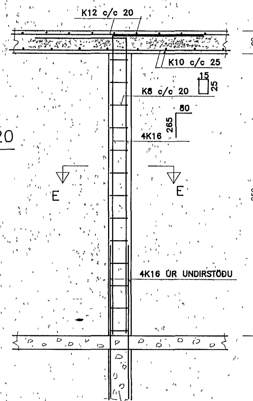
SÚLA S1 1:20
