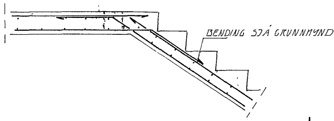
SNID 2. 1:20
