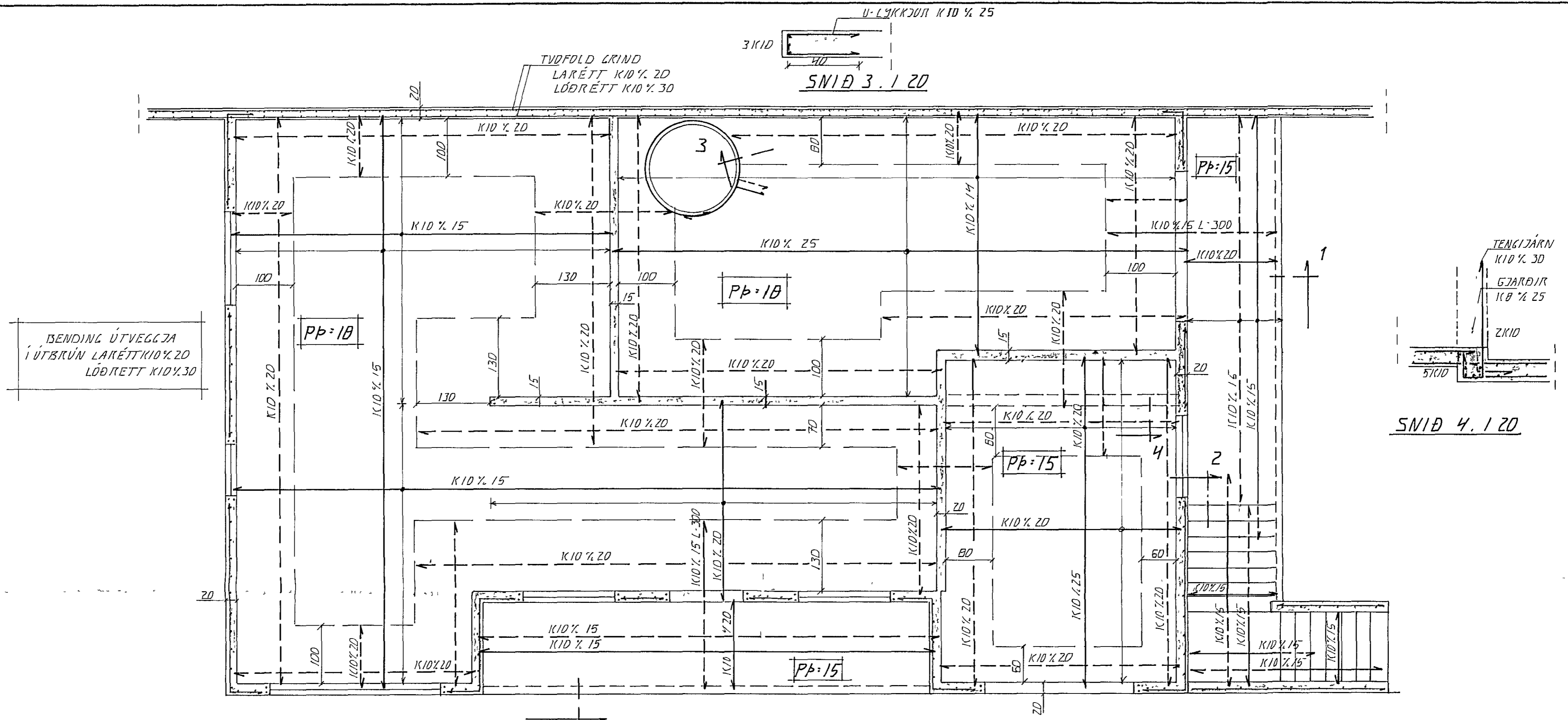
GRUNNMUND 1. HÆÐ. 1:50
