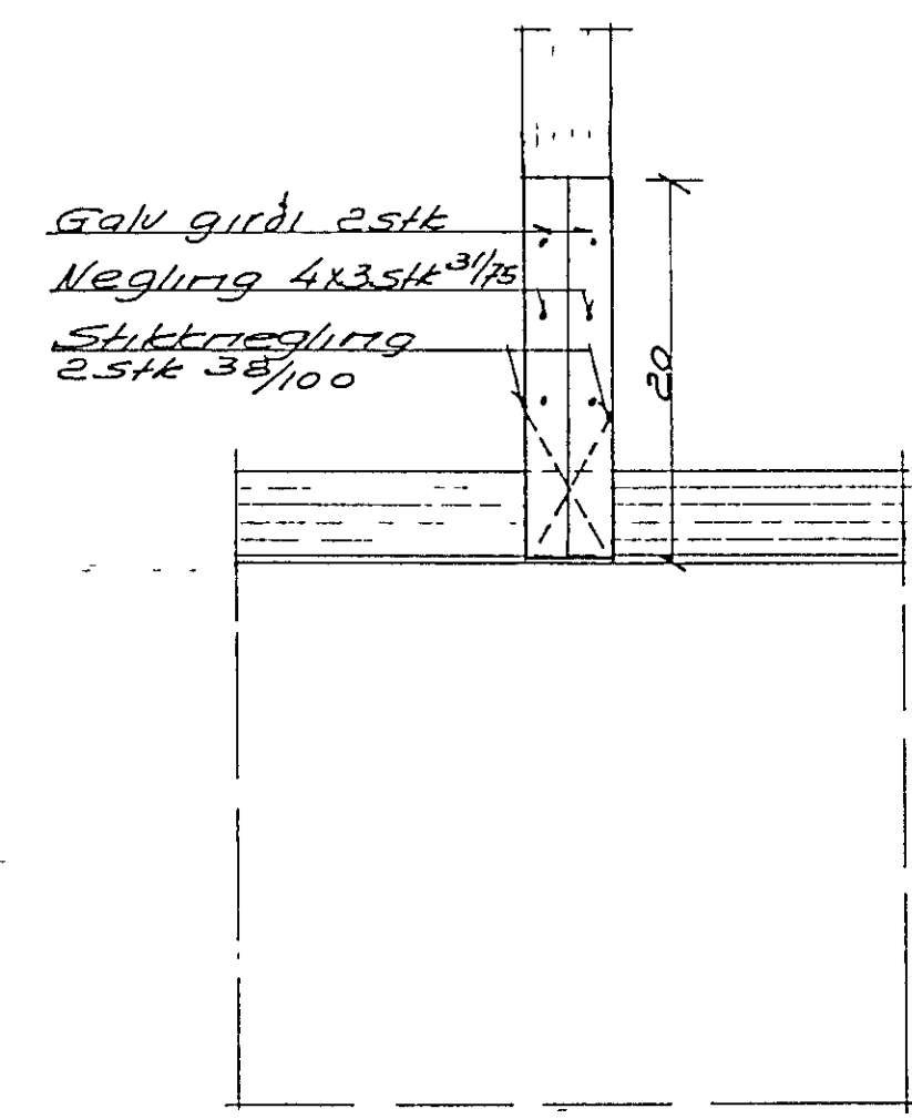
Sníð R2-R2 M1:5 Stoðir milli glugga
