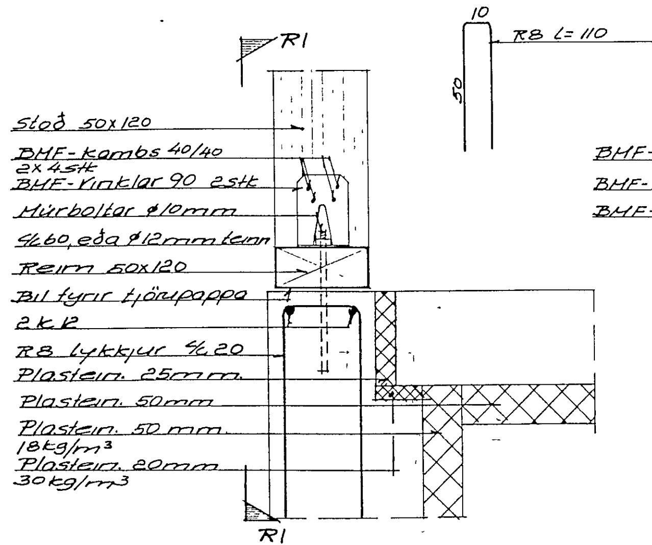
Sníð í sökkul og reim M1:5 Gerd 1
