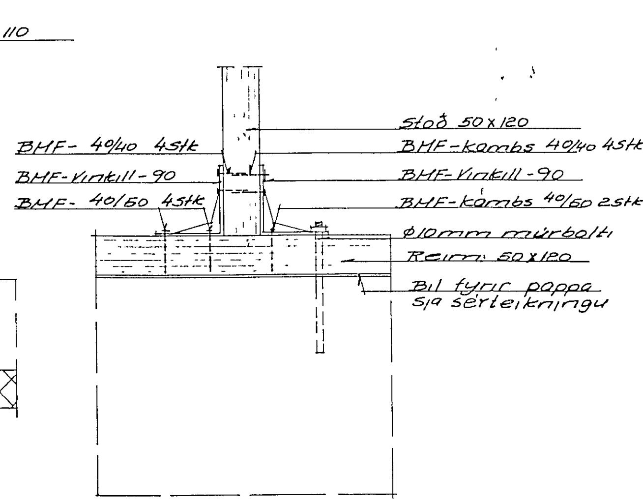
Sníð R1-R1 M1:5 Stoðir við glugga
