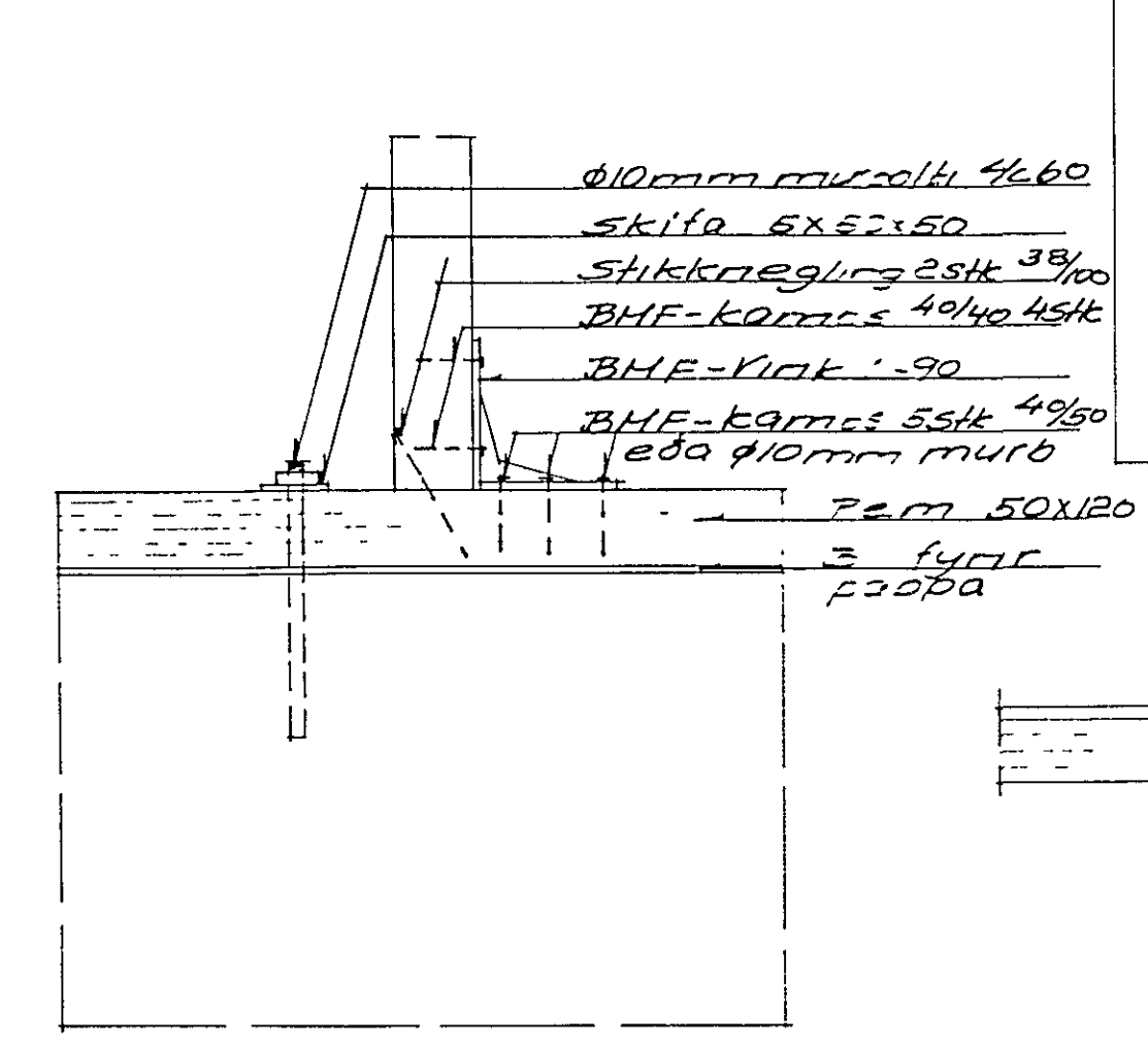
Sníð R1-R1 M1:5 Stoðir milli glugga
