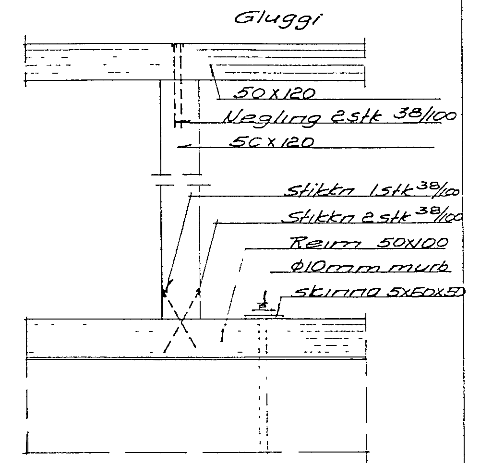
Festing á stoðum undir gluggum.
