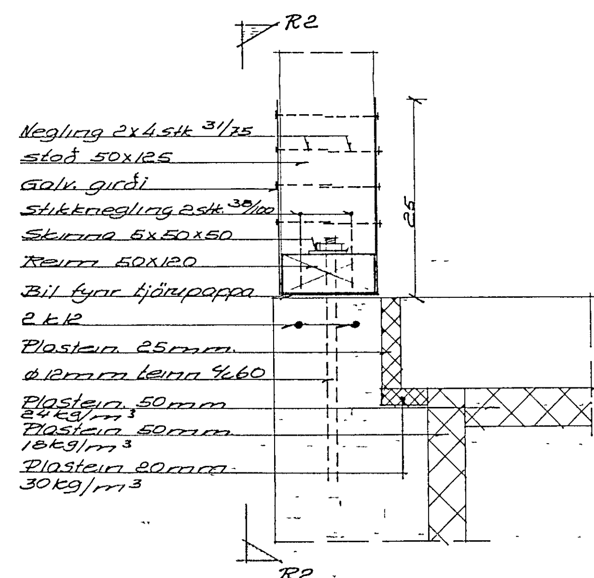
Sníð í sökkul og reim M1:5 Gerd 2
