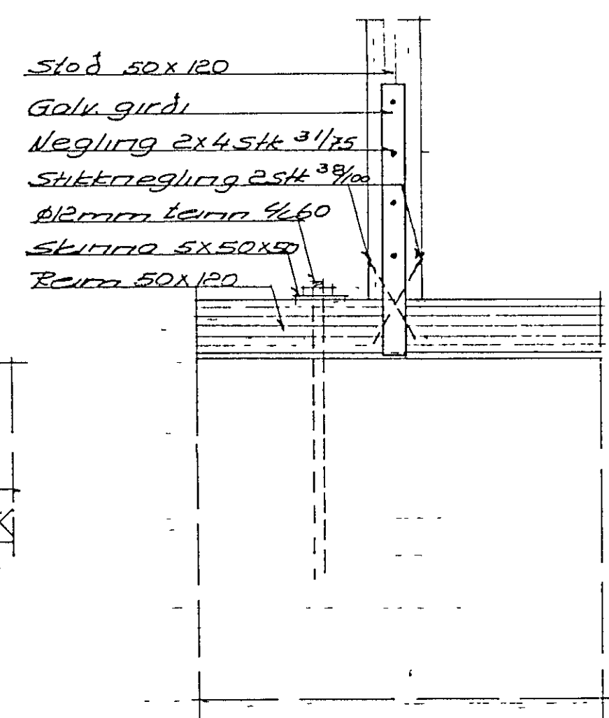
Sníð R2-R2 M1:2 Stoðir milli glugga
