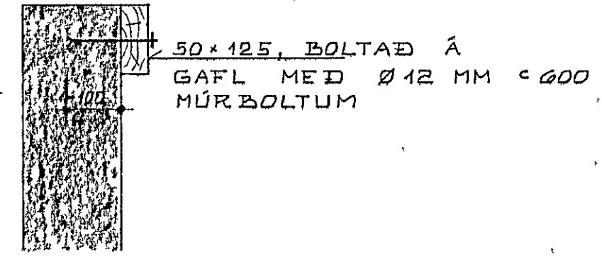
SNÍÐ 3-3 1:10
