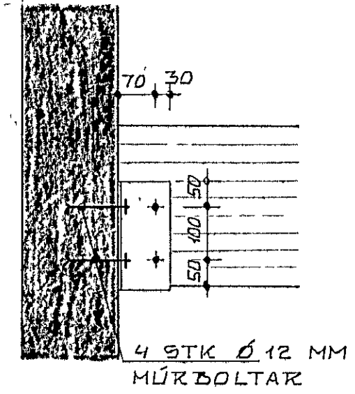
SNIÐ A1-A1 1:10
