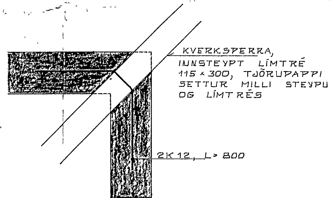
SÉRMYND D 1:10
