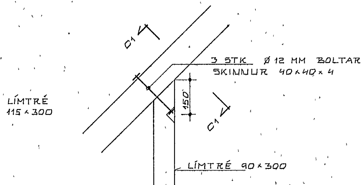
SÉRMYND C 1:10
