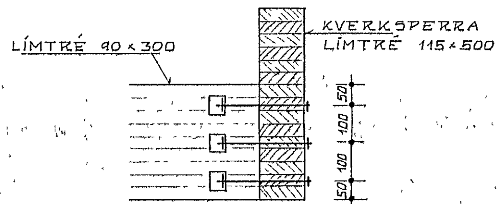
SNIÐ C1-C1 1:10
