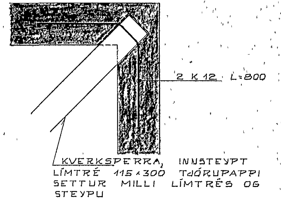
SÉRMYND E 1:10
