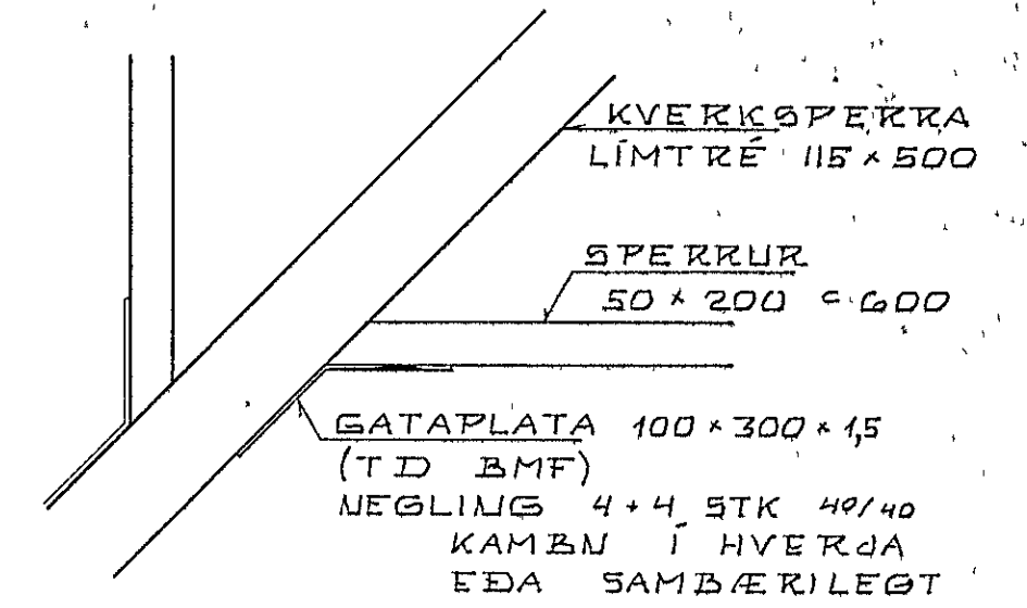
SÉRMYND B 1:10
