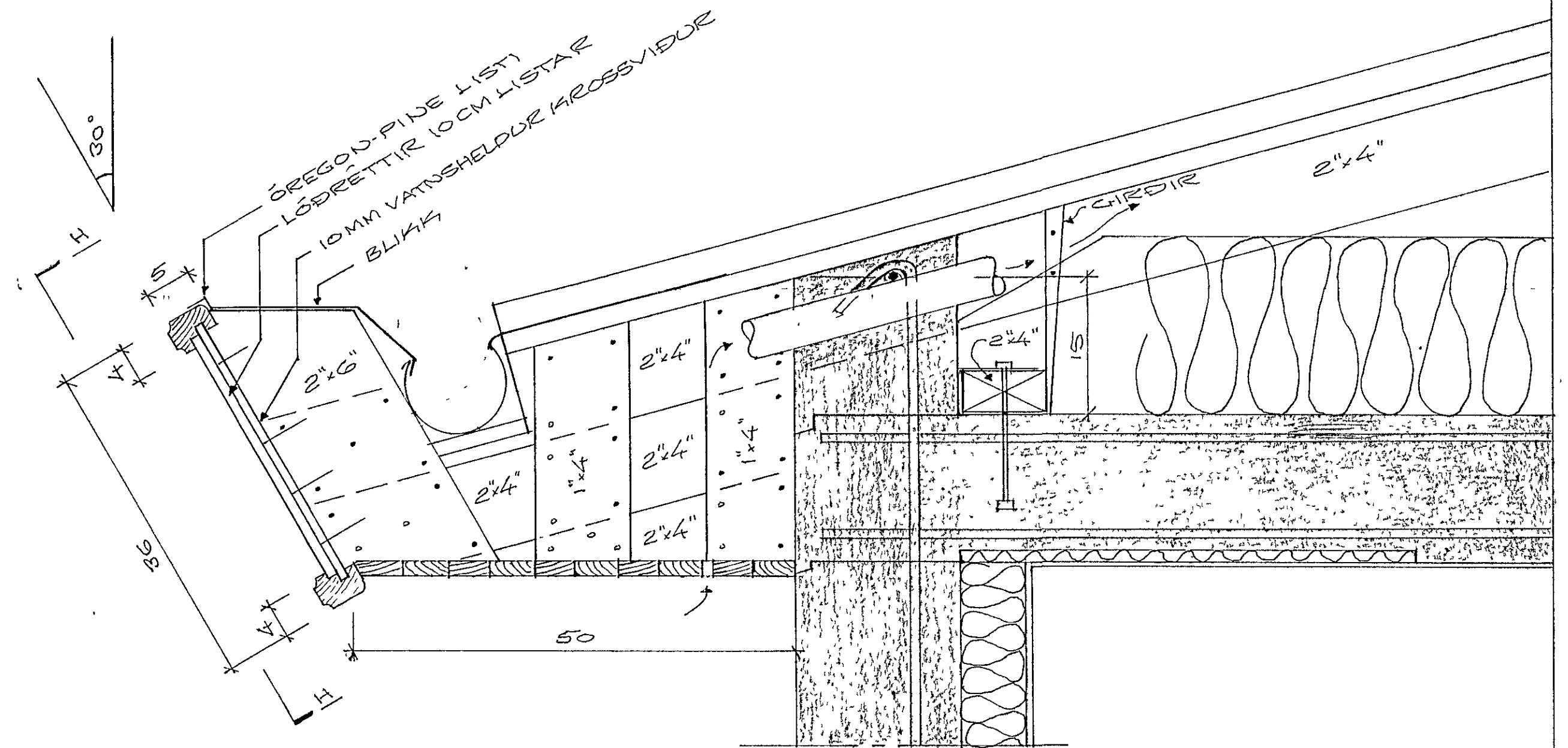
MYND H-H, M=1:5
