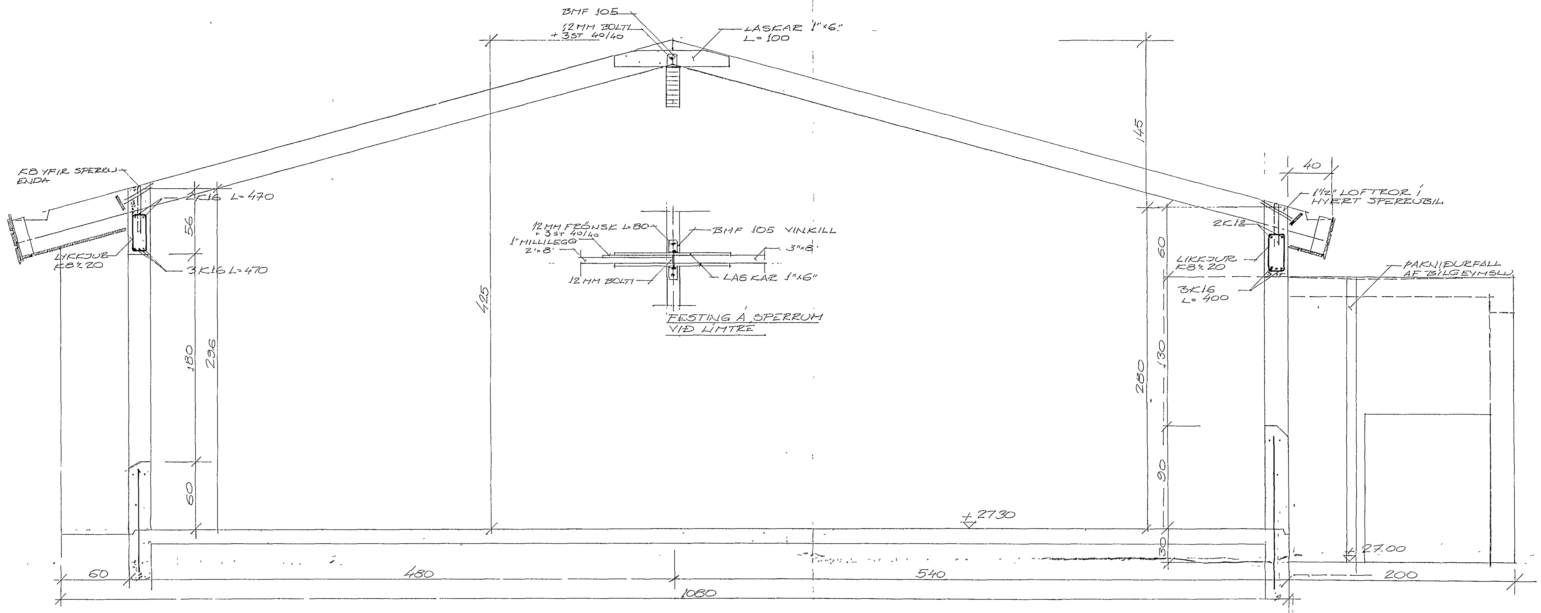
SNID A-A 1:20
