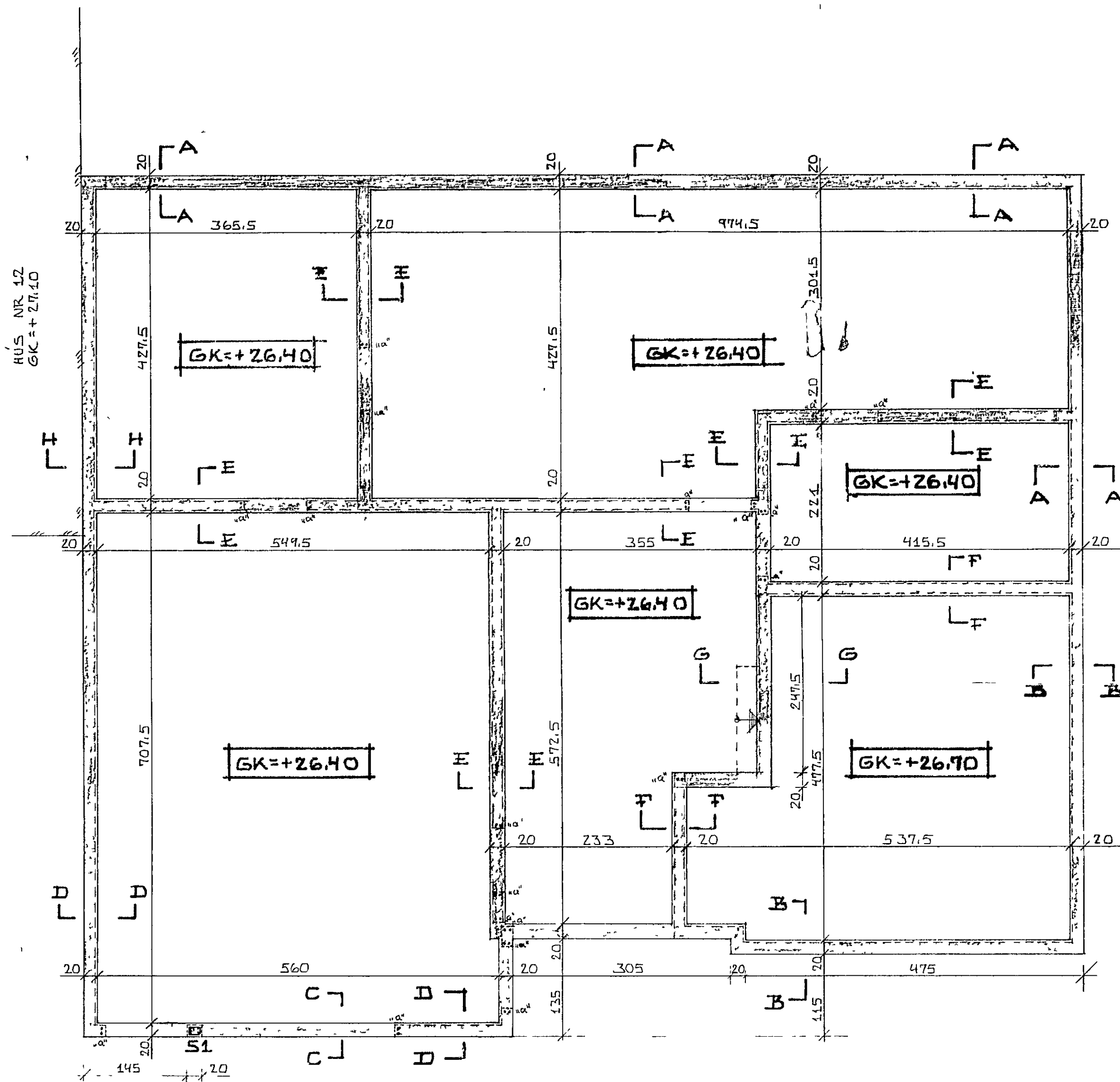
GRUNNMYND 1:50
