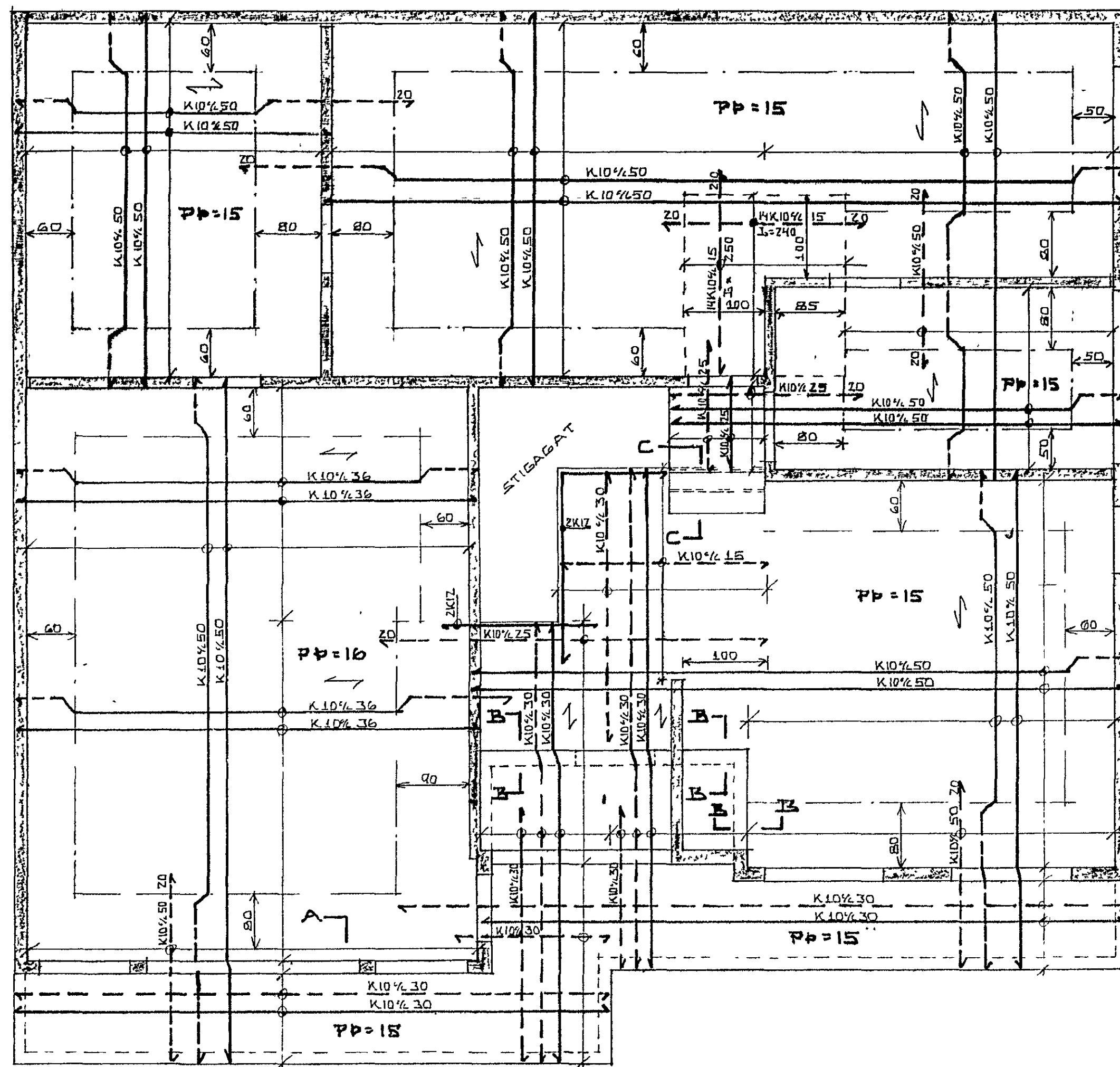
GRUNNMYND 1:50
