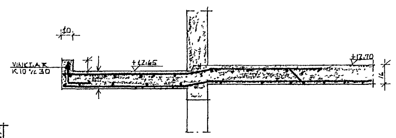
SNID A-A 1:20
