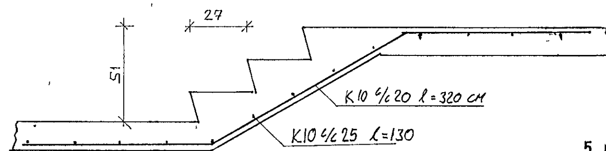
SNEIDING A-A M 1:20
