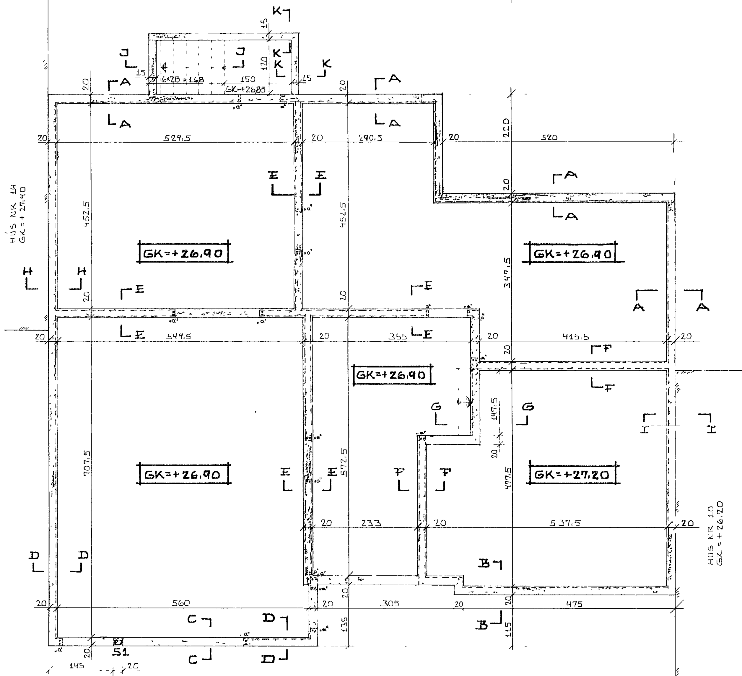
GRUNNMYND 1:50
