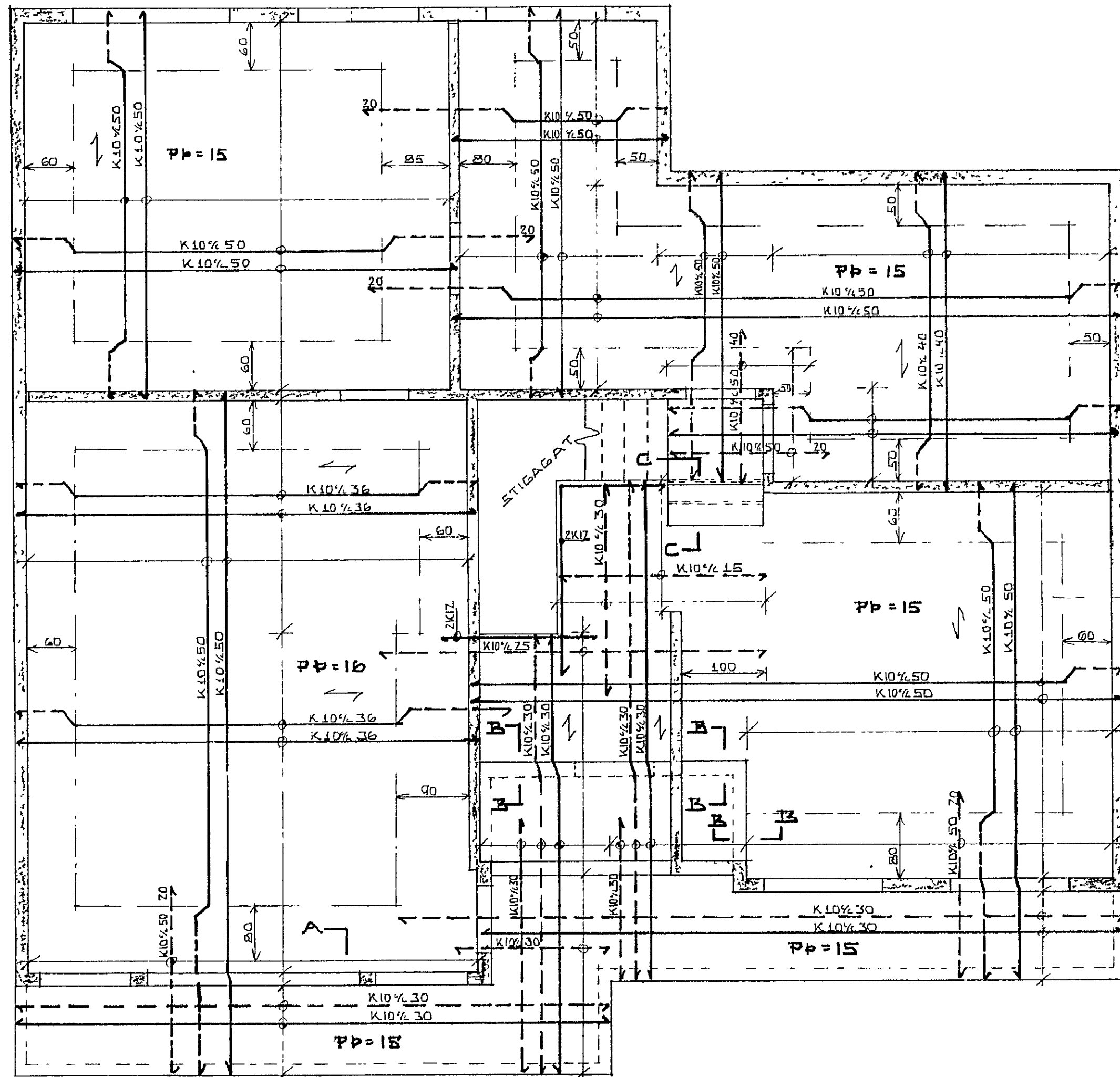
GRUNNMYND 1:50
