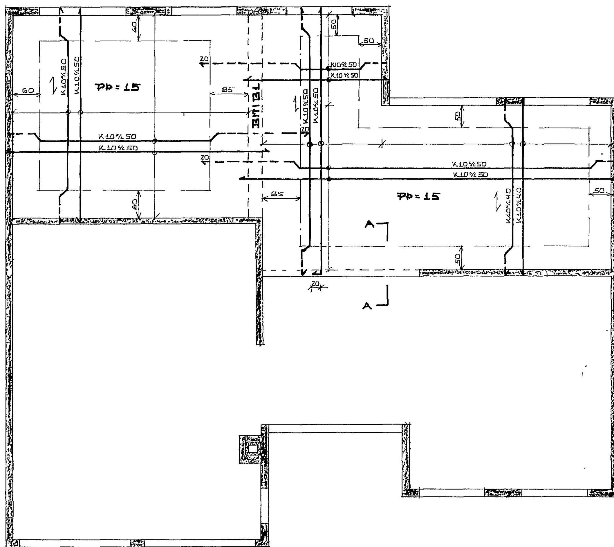
GRUNNMYND 1:50
