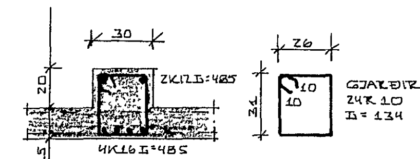
SNİÐ B-B 1:20
