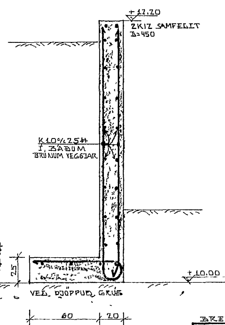
SNID G-G 1:20
