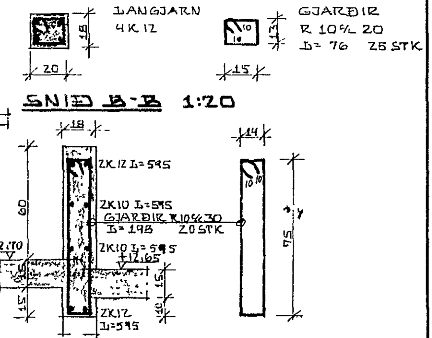
SNID B-B 1:20
