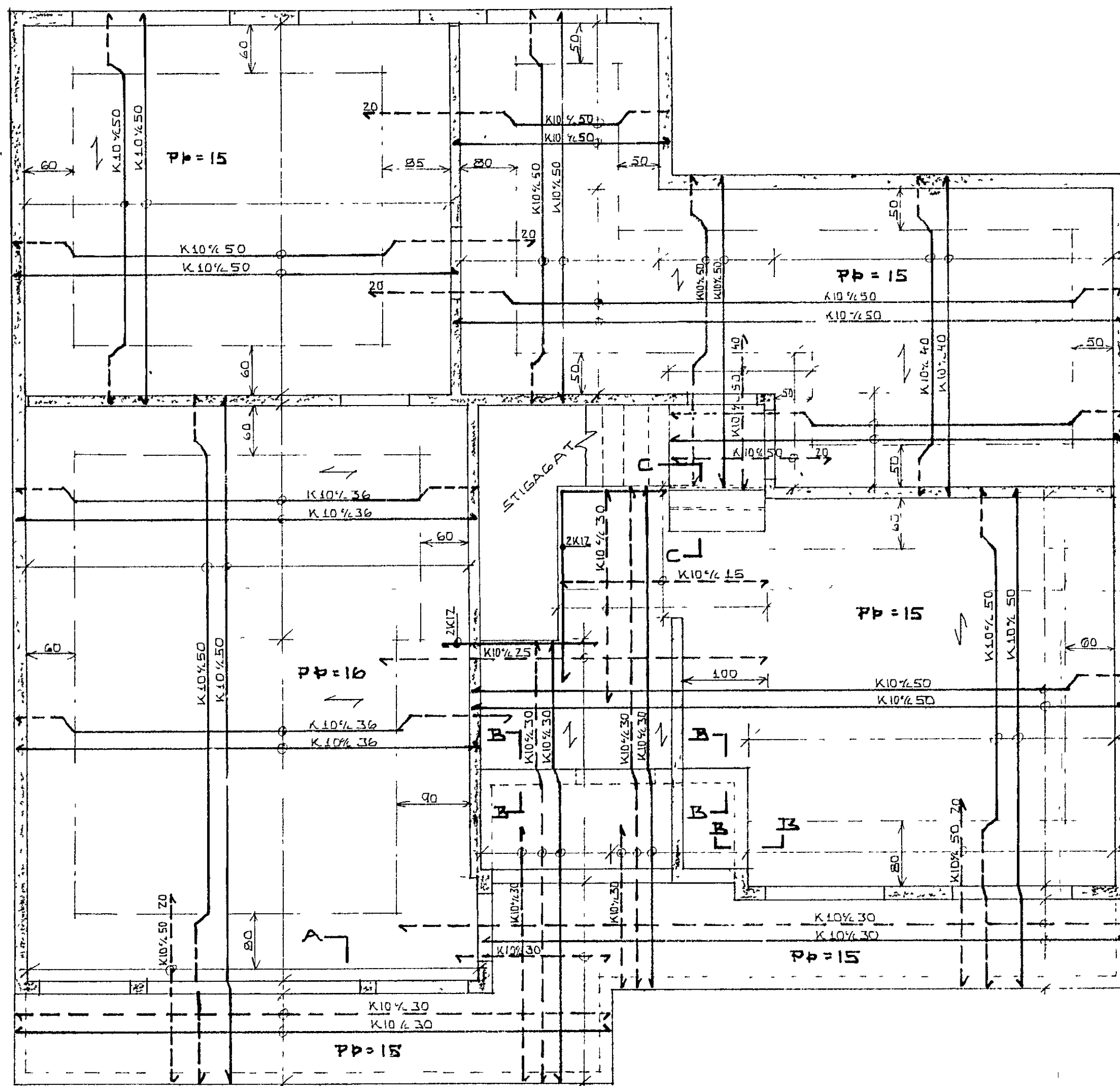
GRUNNMYND 1:50
