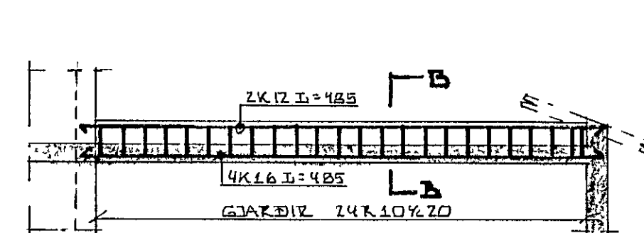
JÁRN Í BÍTA B1 1:50
