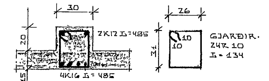
SNID B-B 1:20
