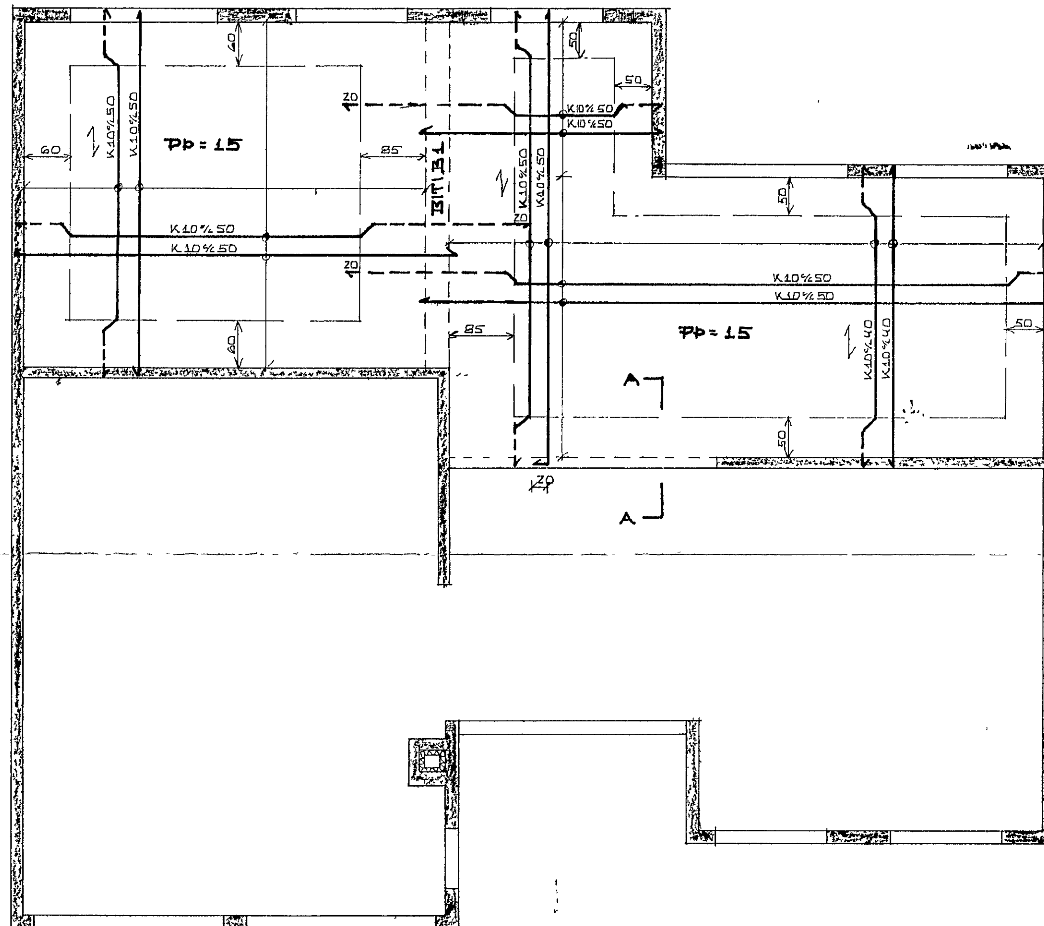
GRUNNMYND 1:50
