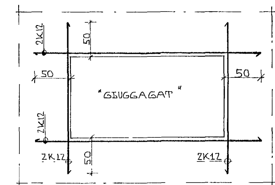
ÞÁRETT SNIÐ
