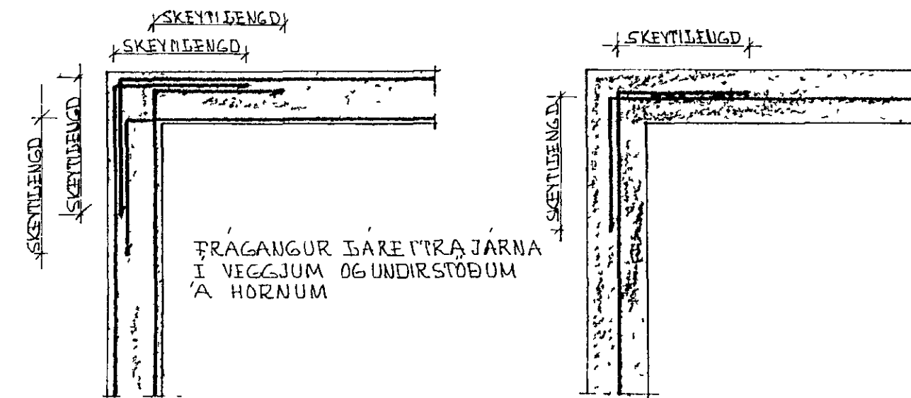
LÁRETT SNIÐ
