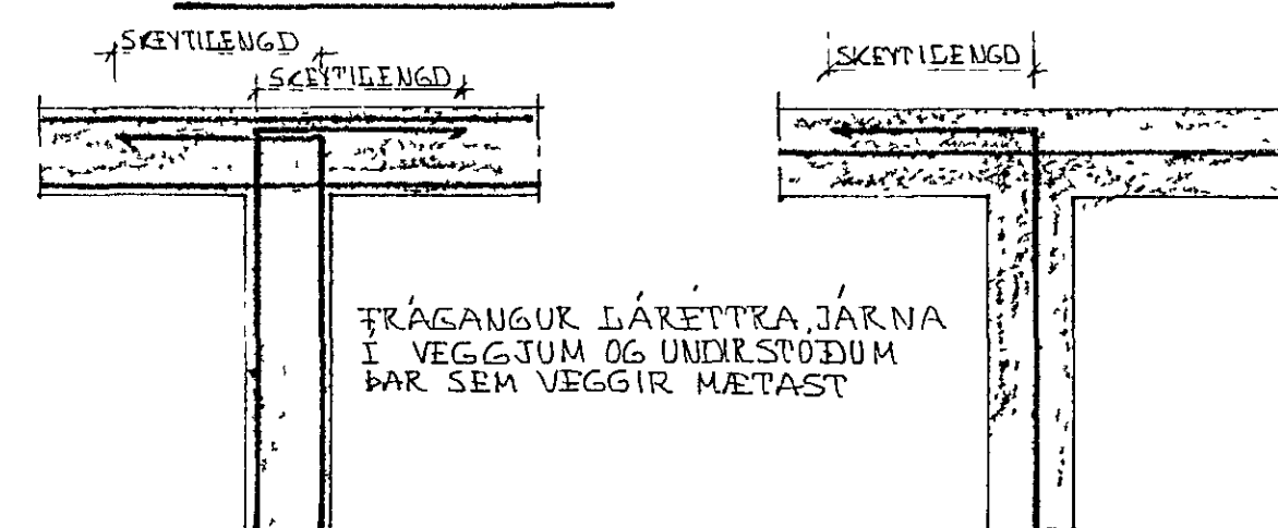
ÞÁRETT SNIÐ
