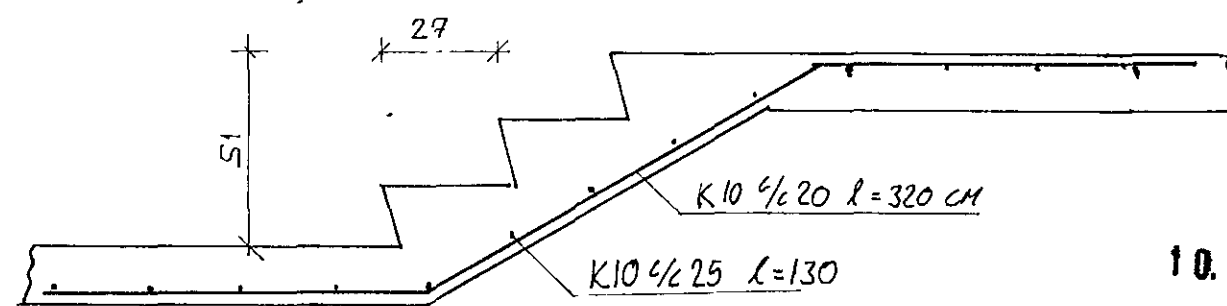
SNEIÐING A-A M 1:20
