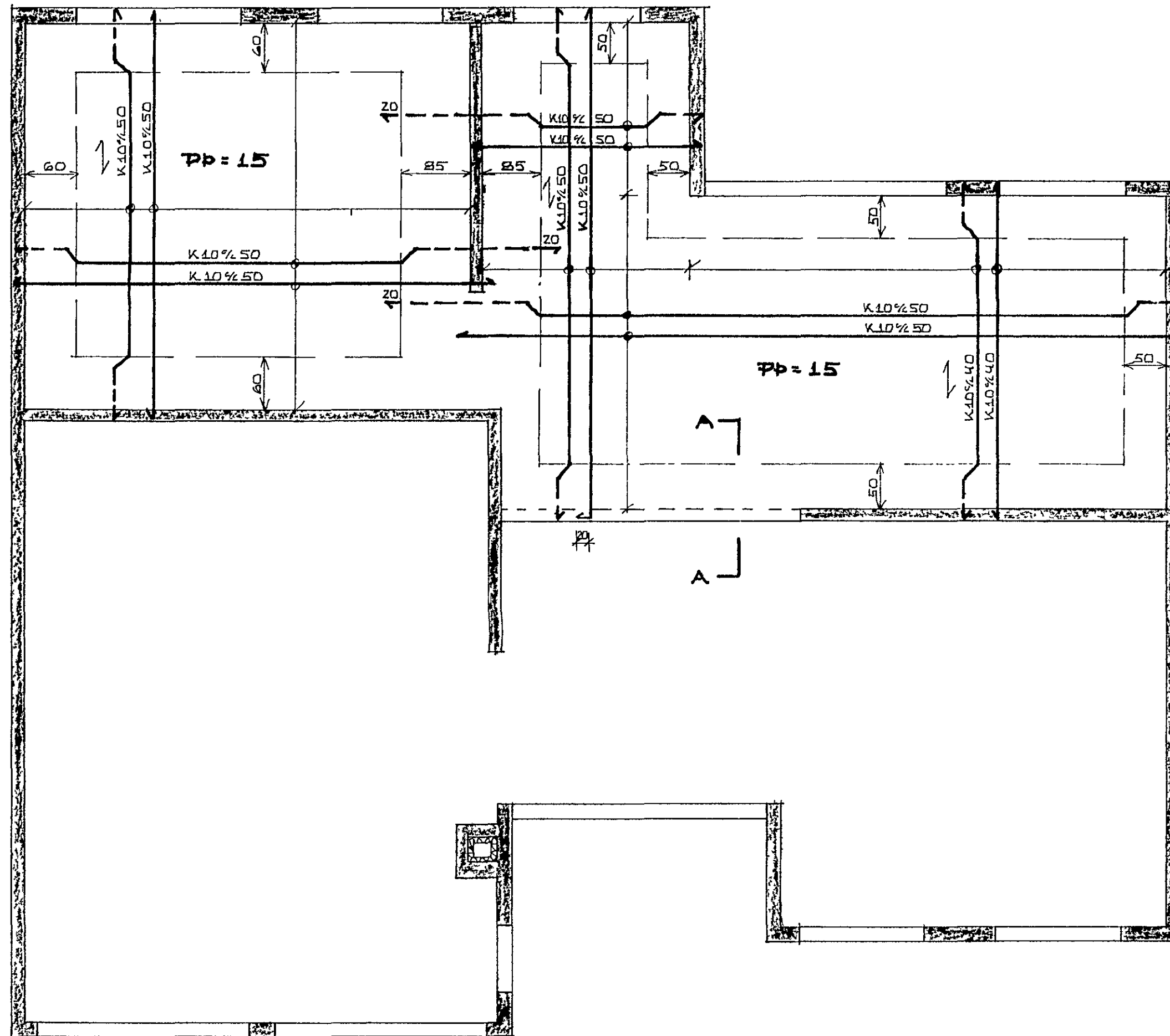
GRUNNMYND 1:50
