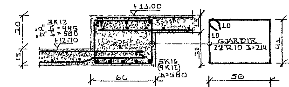
SNID D-D 1:20
