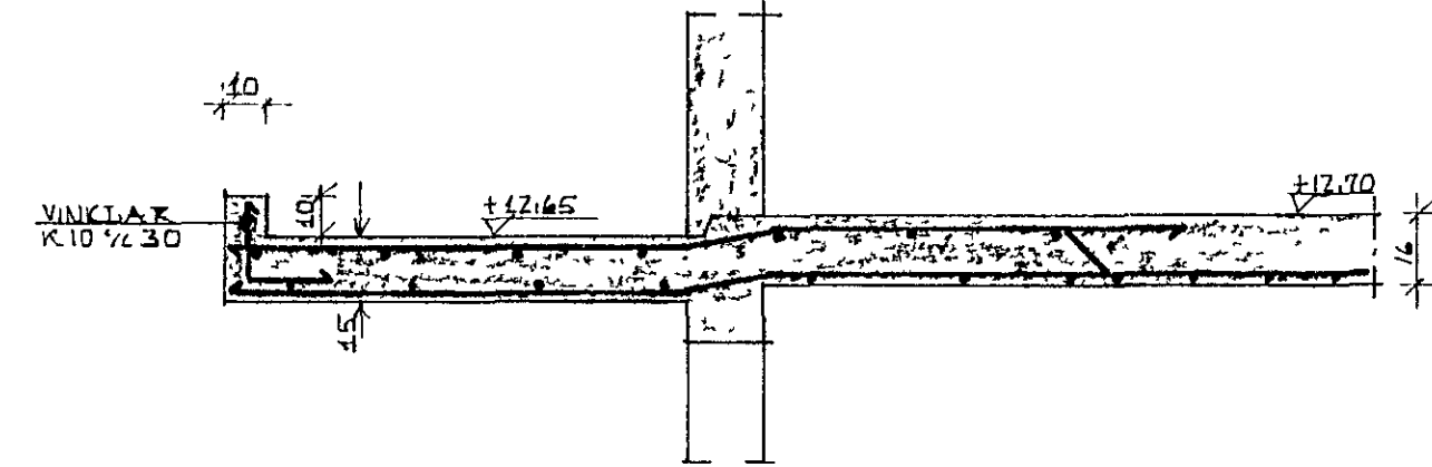
SNID A-A 1:20
