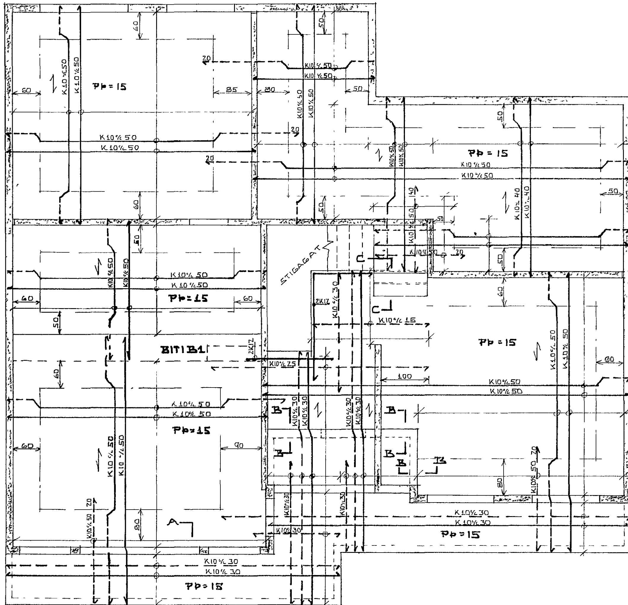
GRUNNMYND 1:50
