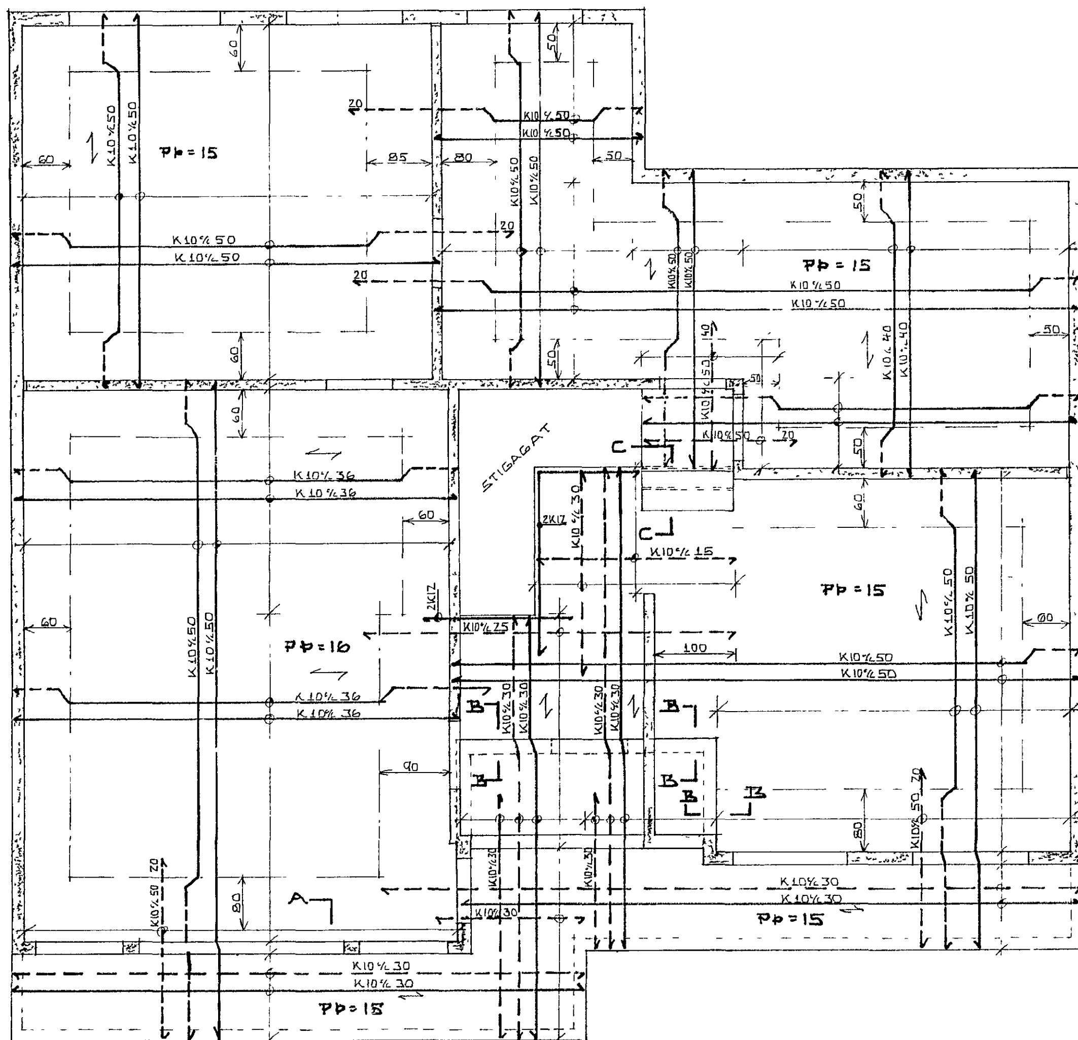
GRUNNMYND 1:50
