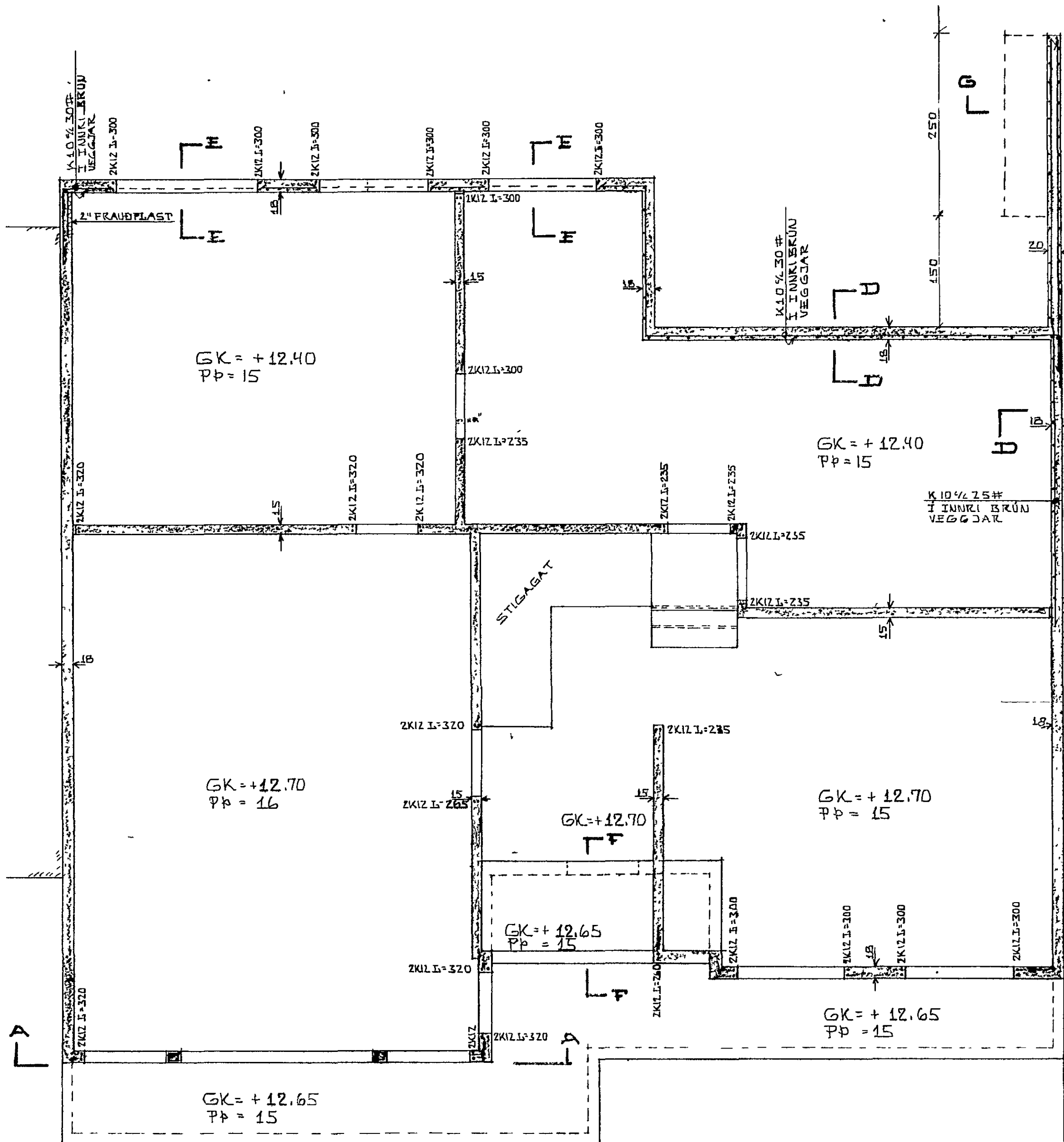
GRUNNMYND 1:50
