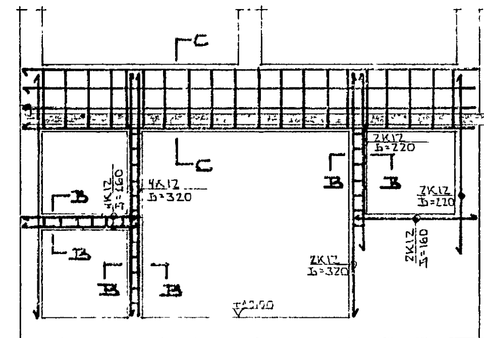
SNID A-A 1:50
