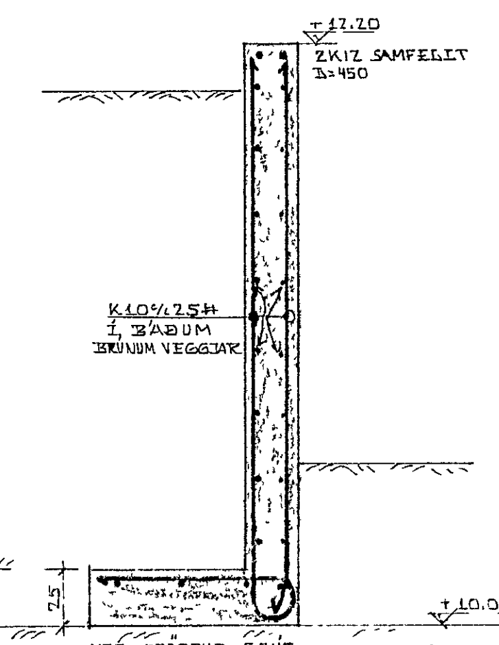
SNID G-G 1:20
