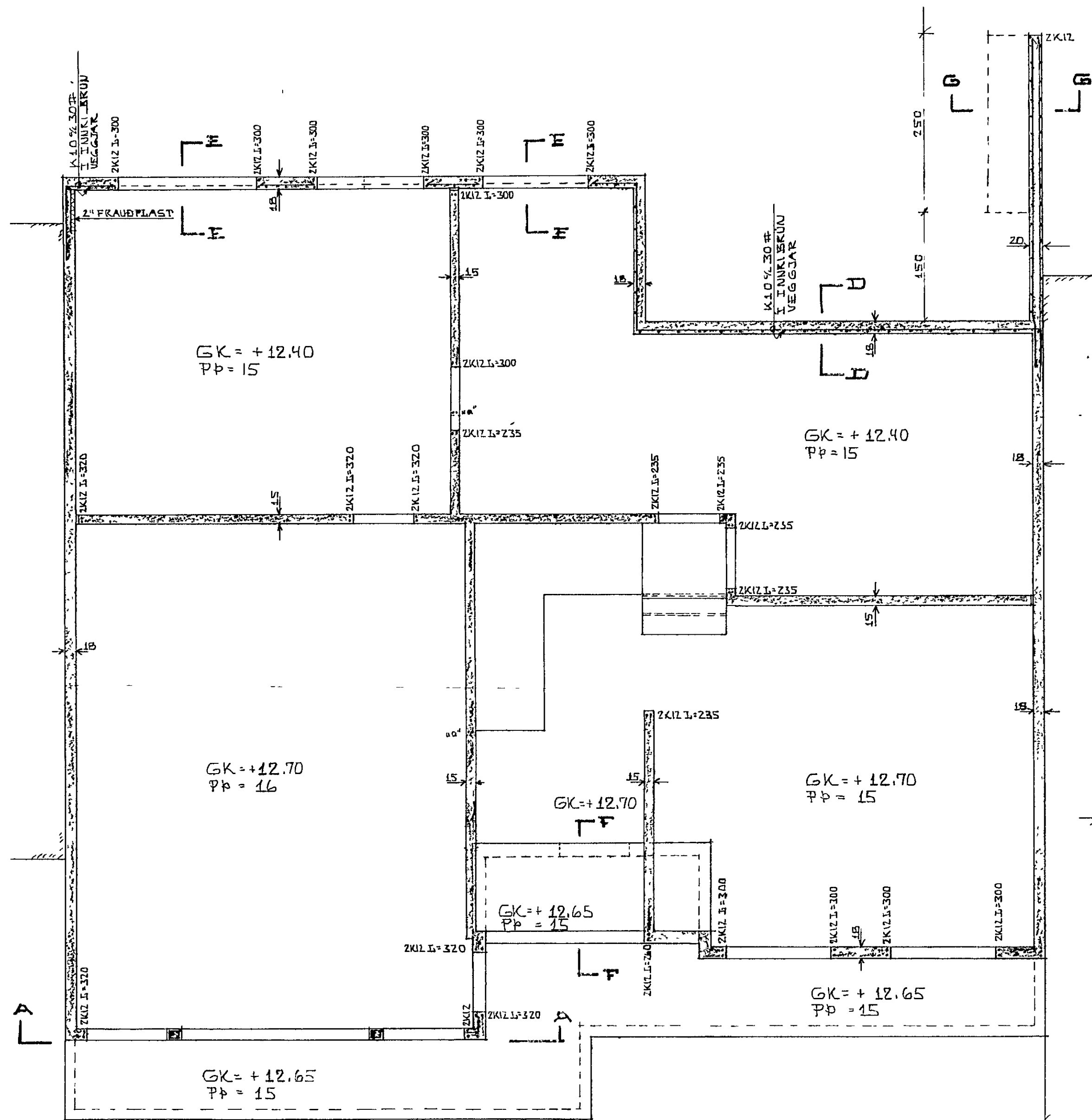
GRUNNMYND 1:50
