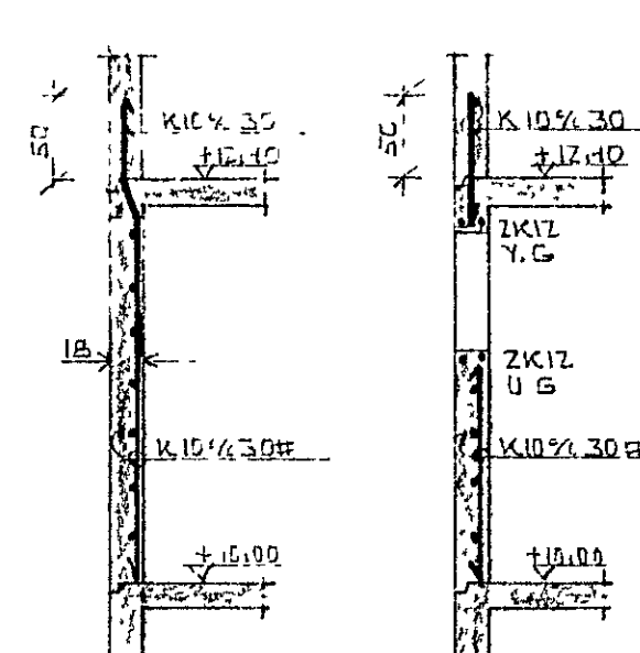
SNID D-D 1:50
