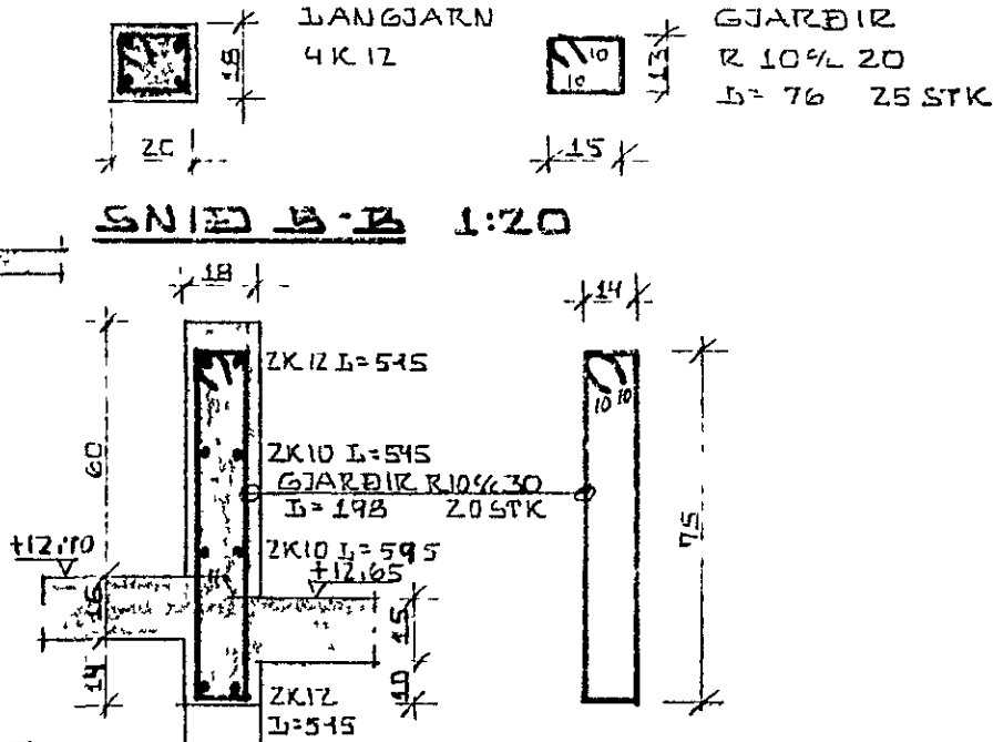
SNID B-B 1:20
