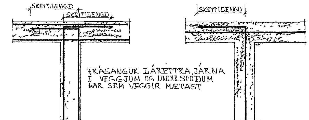
LÁRETT SNIÐ
