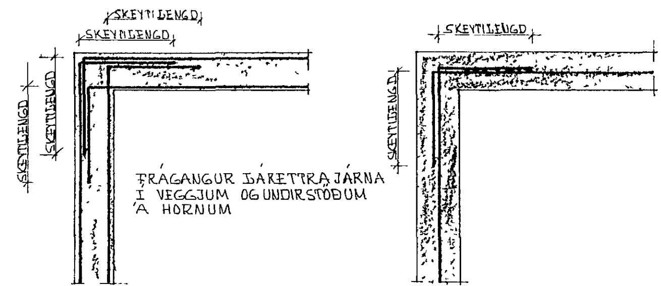
LÁRETT SNIÐ
