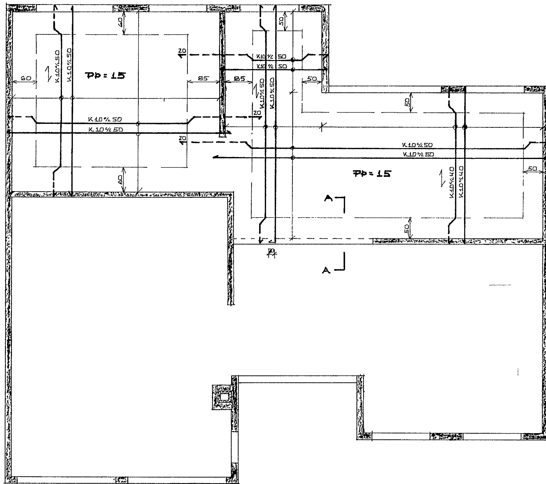
GRUNNMYND 1:50
