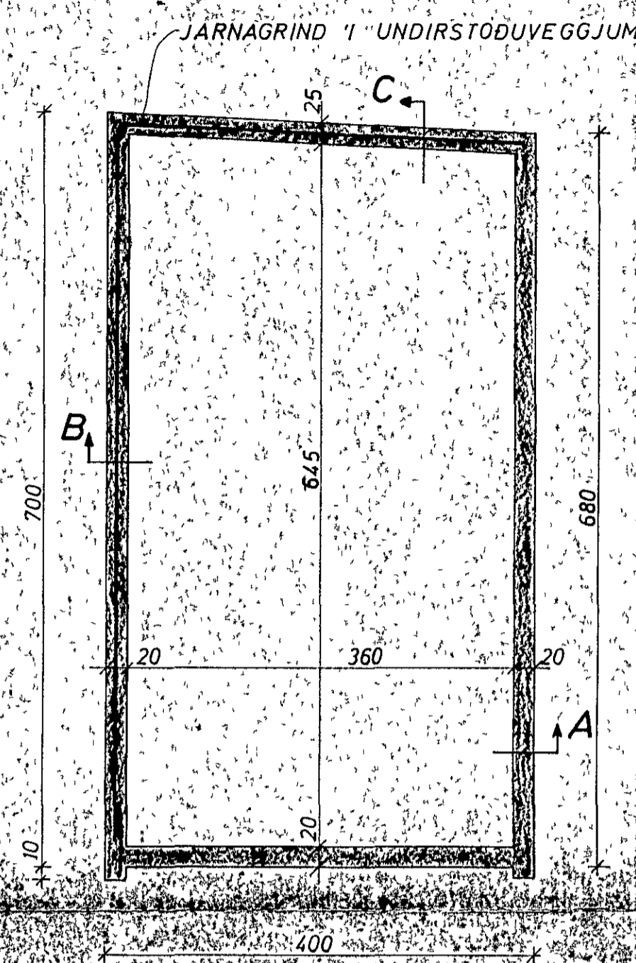
UNDIRSTÖÐUR
