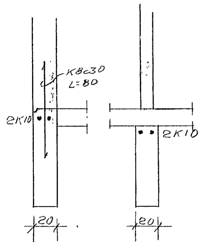
SNEIÞINGIÐ 1:20
