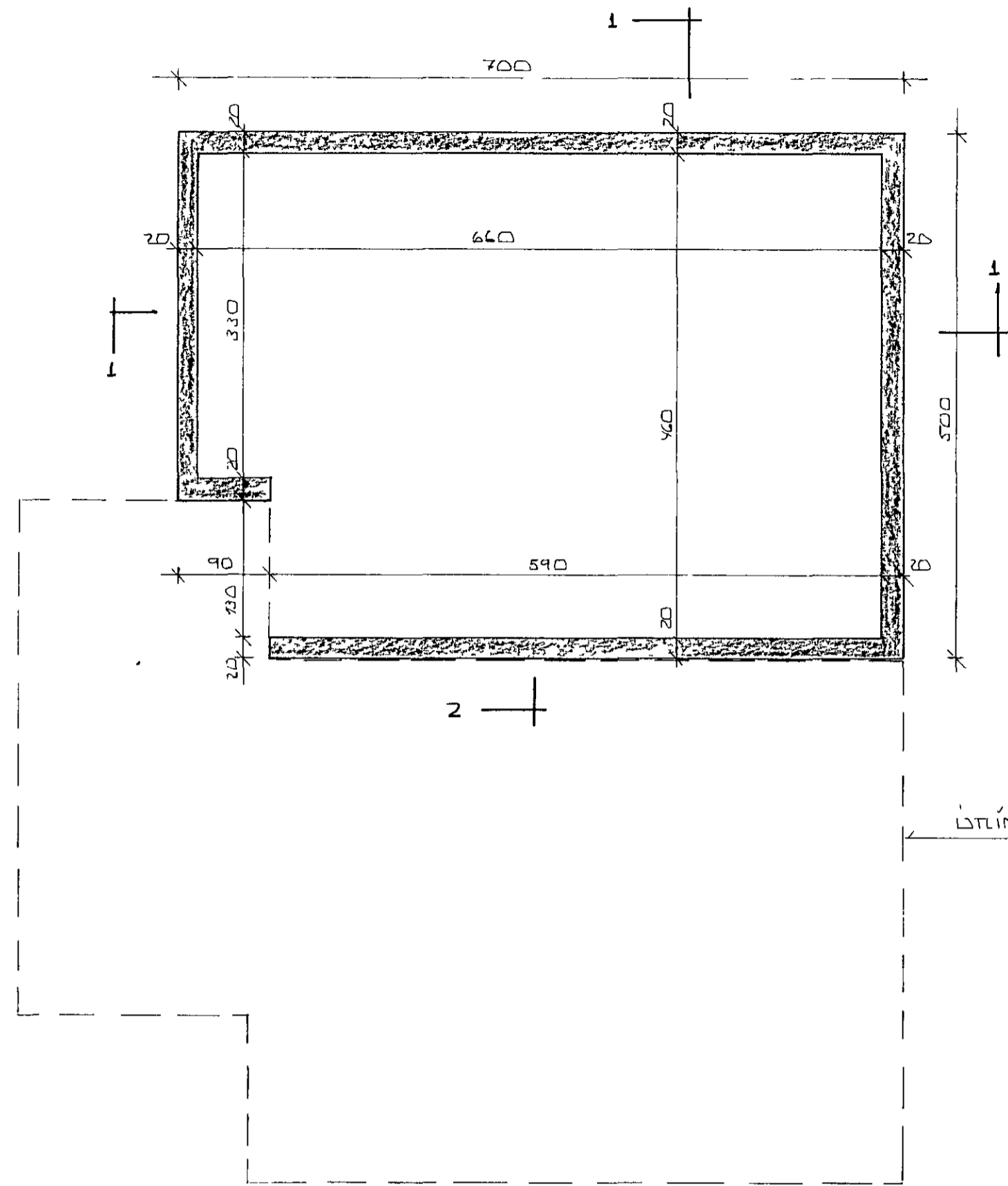
GRUNNMYND ~ 1:50
