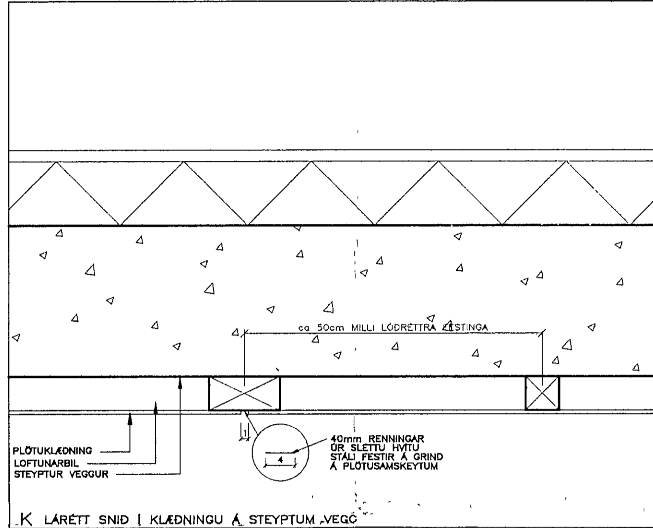
K LÁRETT SNID I KLÆDNINGU Á STEYPTUM VEGG
