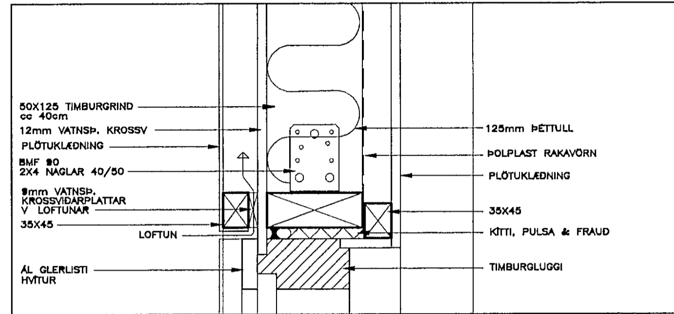
D LÓDRÉTT SNID VID EFRI BRÚN GLUGGA
