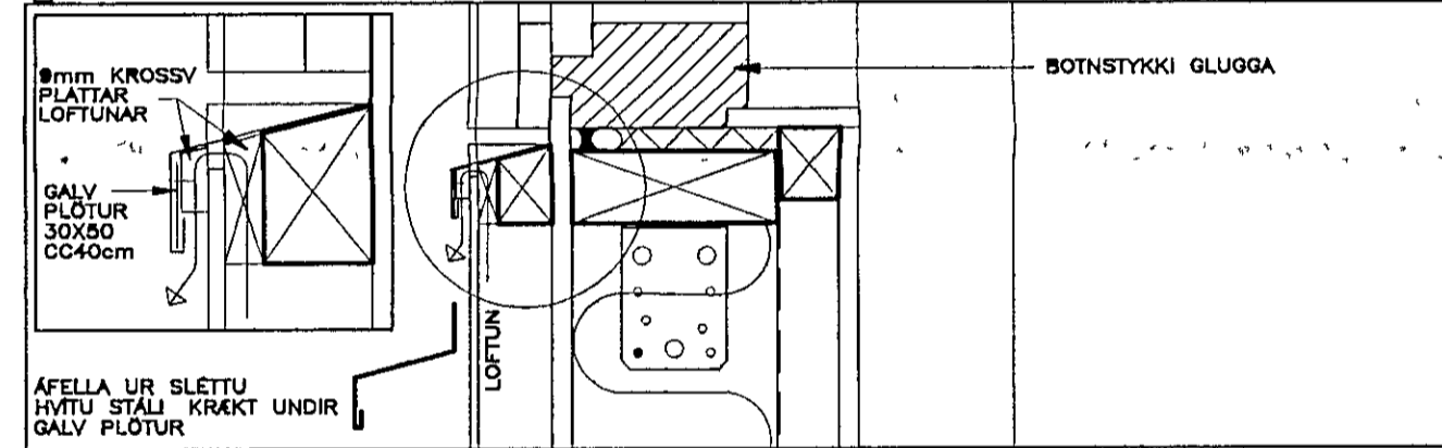
F LÓDRÉTT SNID VID NEDRI BRUN GLUGGA
