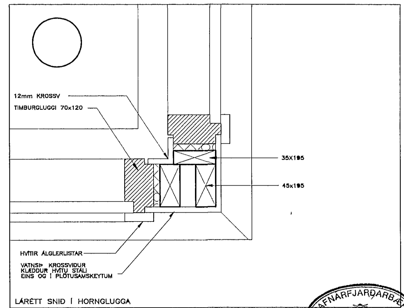
M LÁRETT SNID I KLÆDNINGU Á STEYPTUM VEGG VID UTHORN
