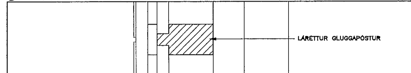
E LÓDRÉTT SNID I LÁRETTAN GLUGGAÞÓST
