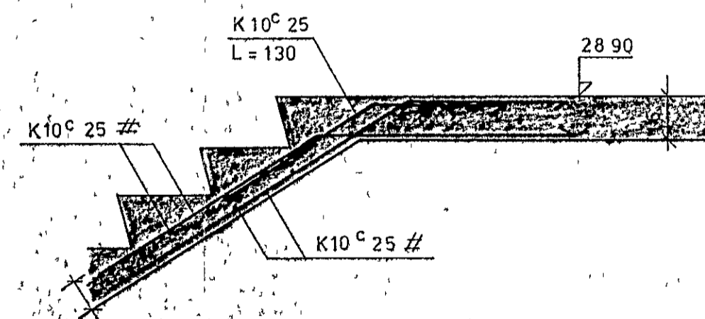
SNID 8-8 1:20 NR. 9
