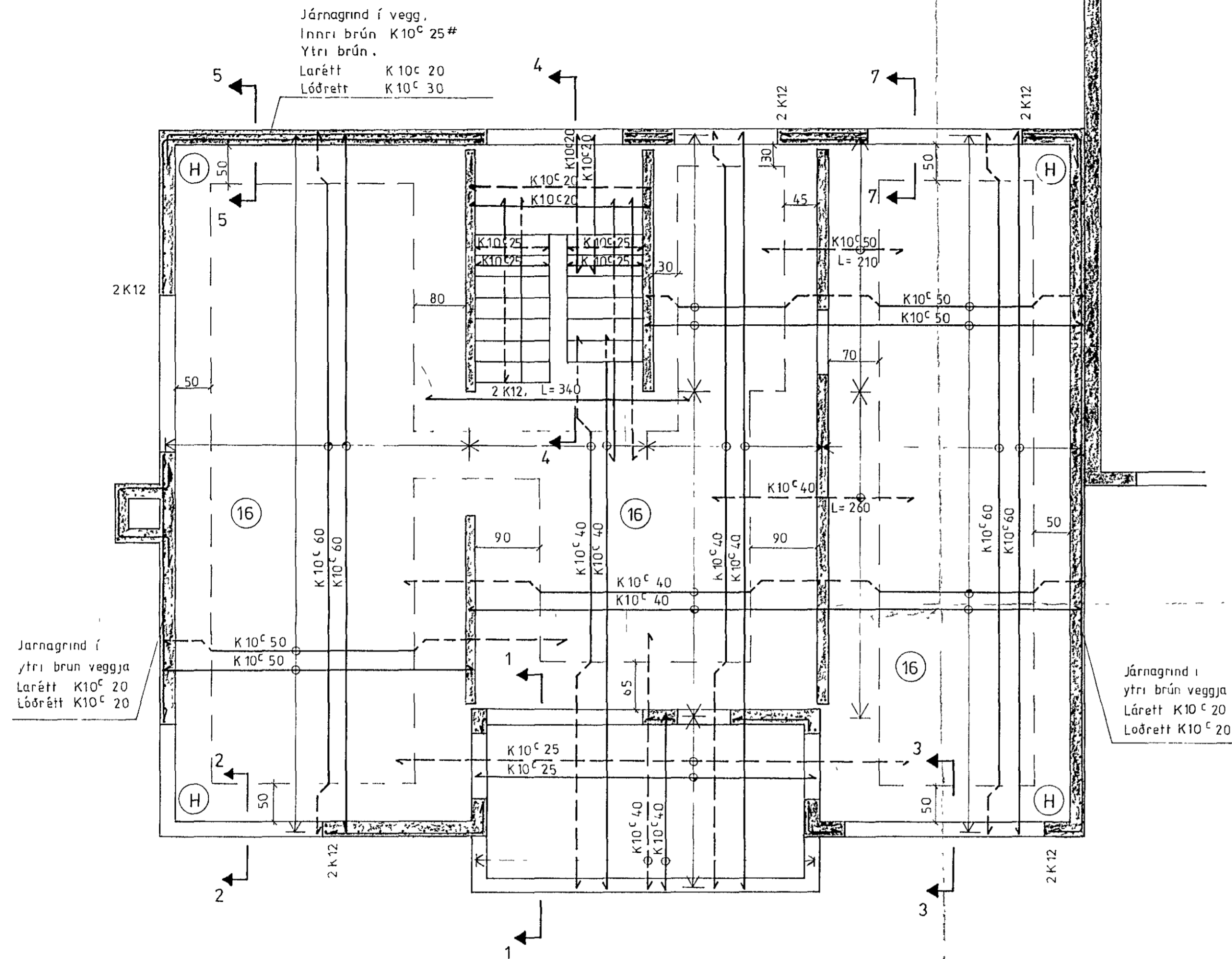
GRUNNMYND 1:50
