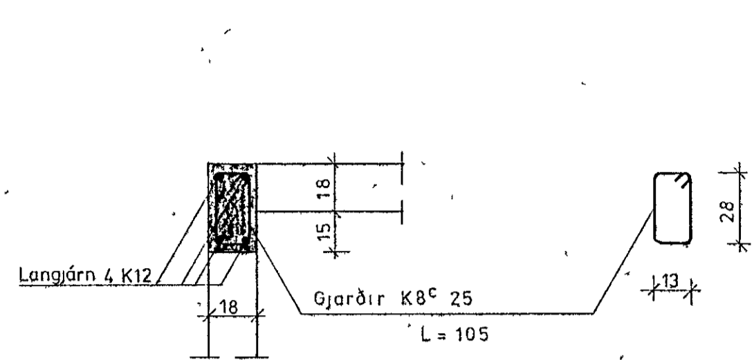
SÚLA S1 1:20
