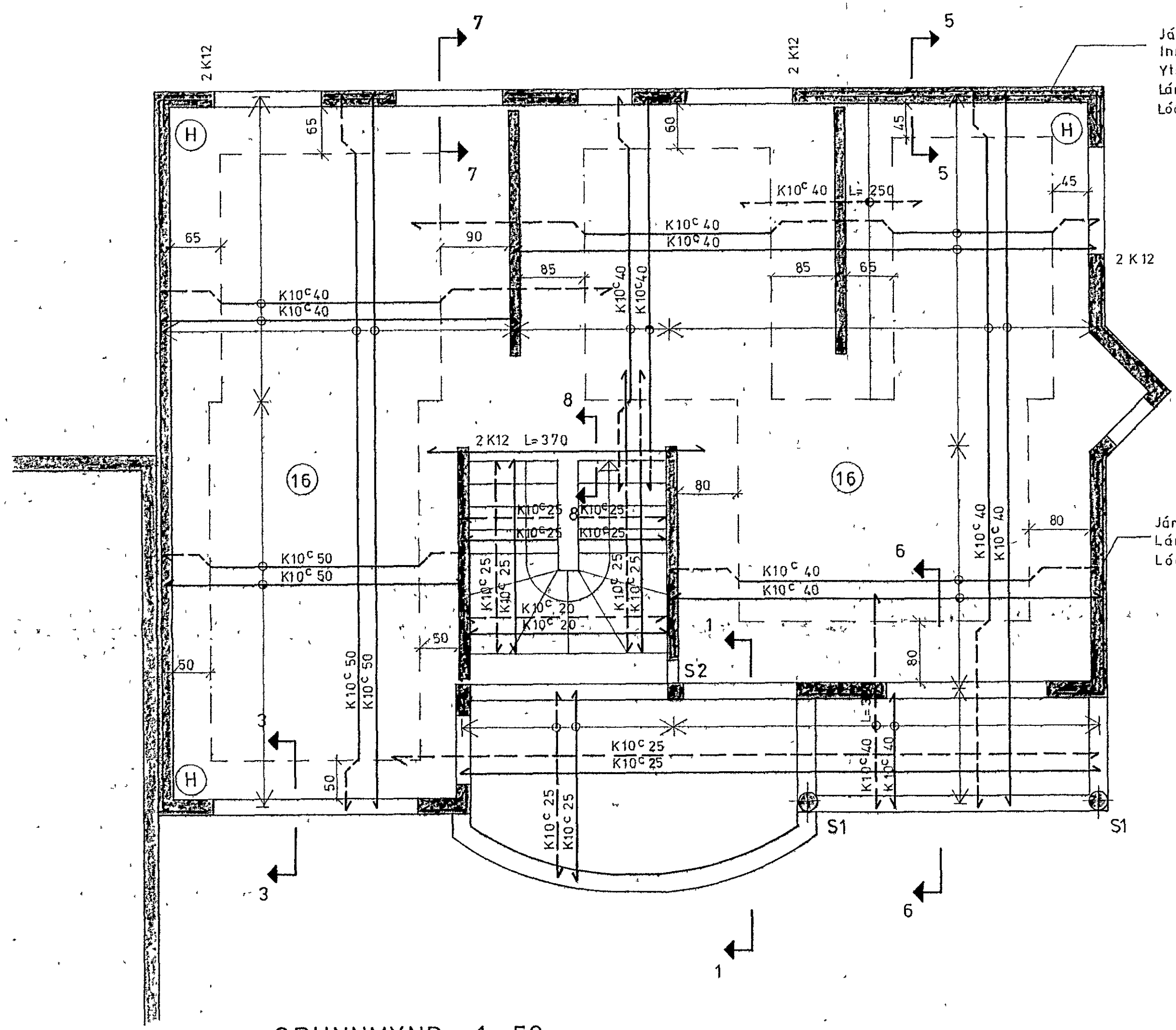
GRUNNMYND 1:50
