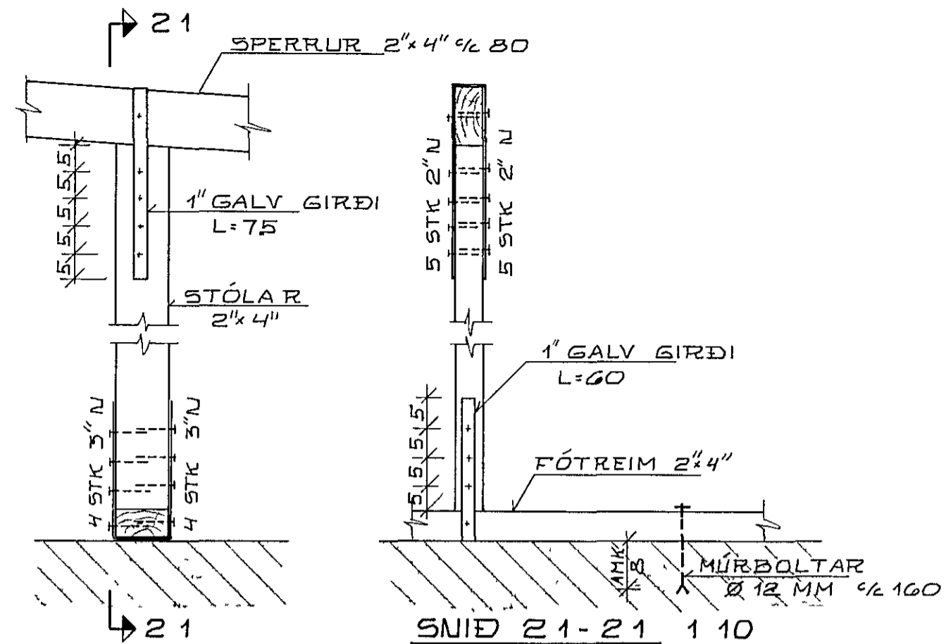
SÉRMYND 2 1 10
