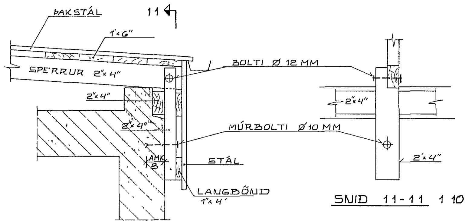
SÉRMYND 1 1 10
