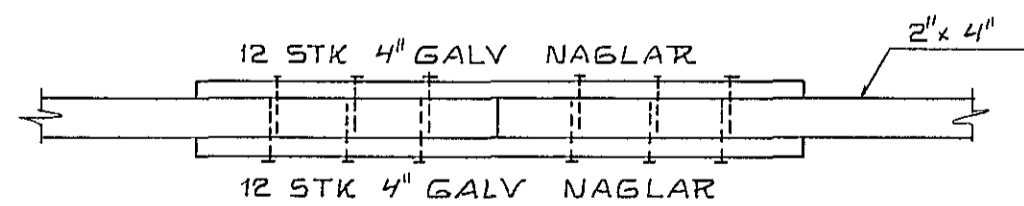
SNIÐ 41-41 1.10
