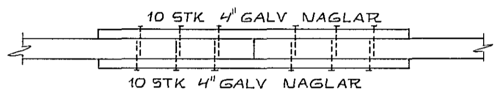
SNIÐ 31-31 1 10
