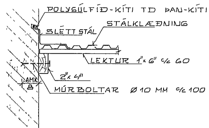
SNIÐ B-B 1 10
