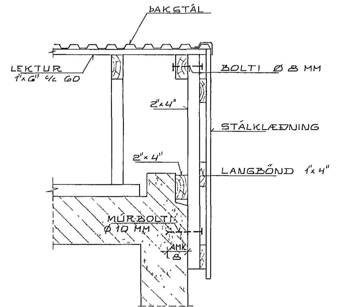
SNIÐ C-C 1 10
