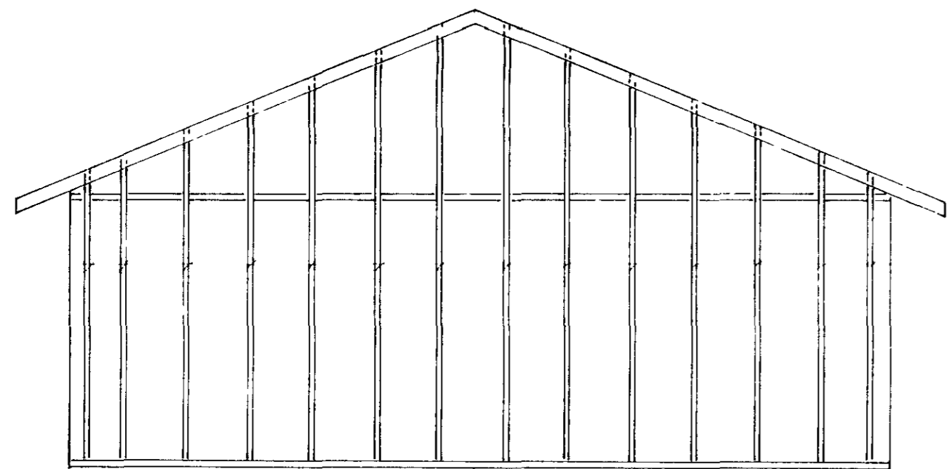
ÁSYND NORÐURGAFL . 1 50
