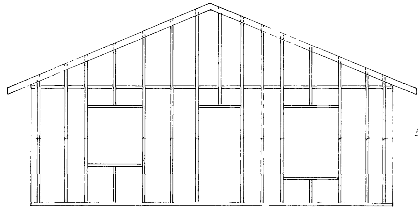
ÁSYND SUÐURGAFL . 1 50
