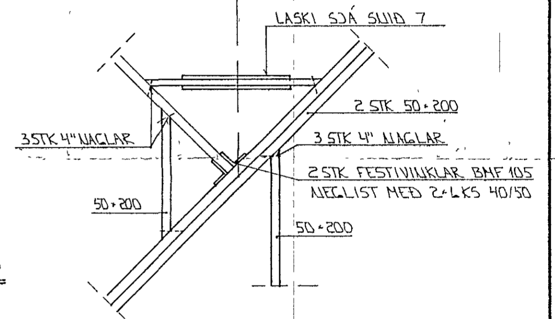
SÉRMYND A 1:20
