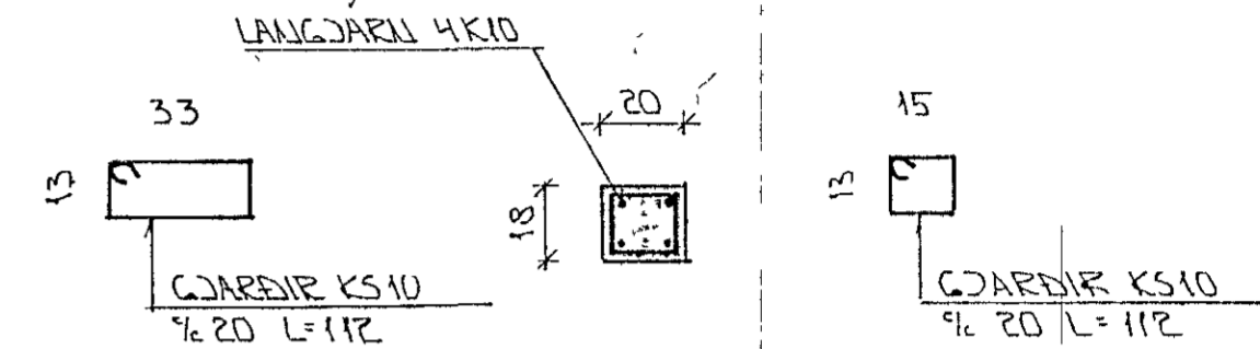
SÚLA S2 1:20
