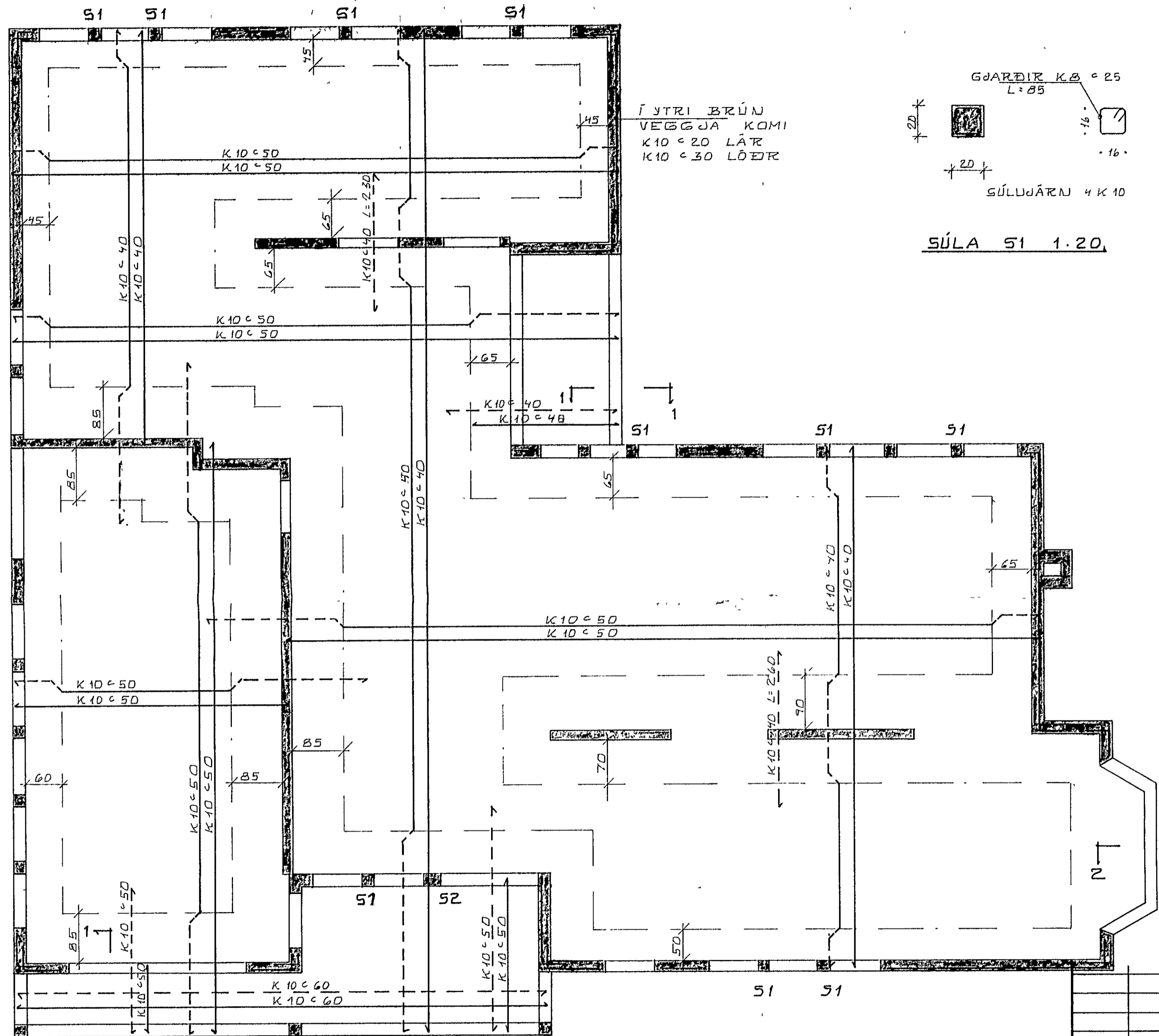
GRUNNMYND 1:50
