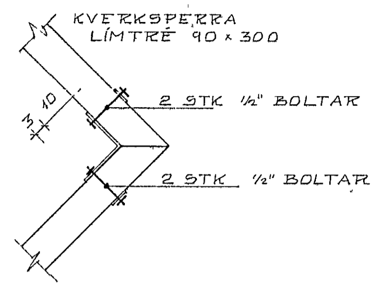
SÉRMYND I 1:10
