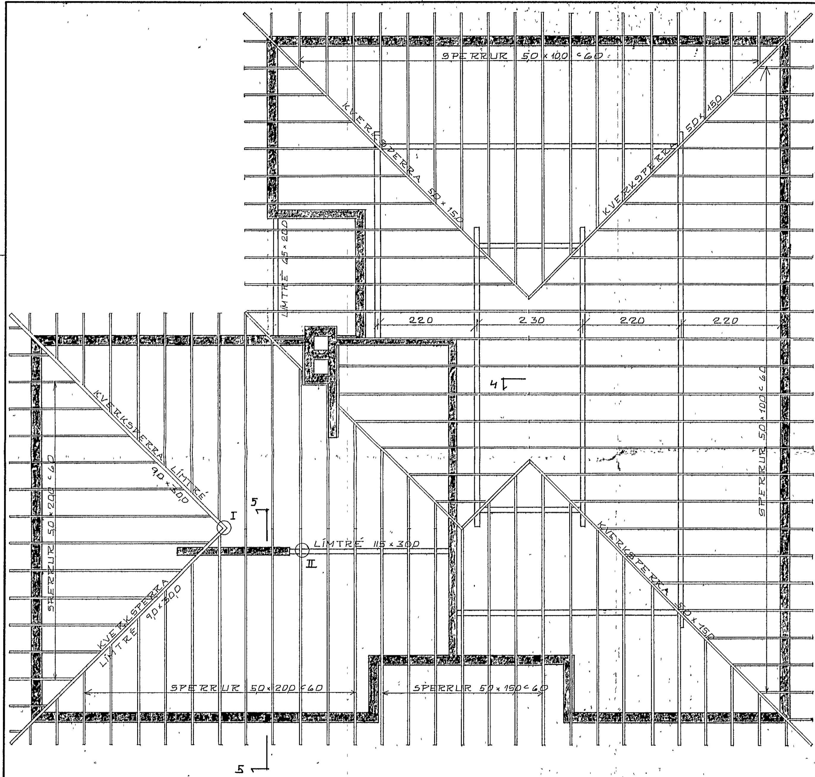
GRUNNMYND 1:50
