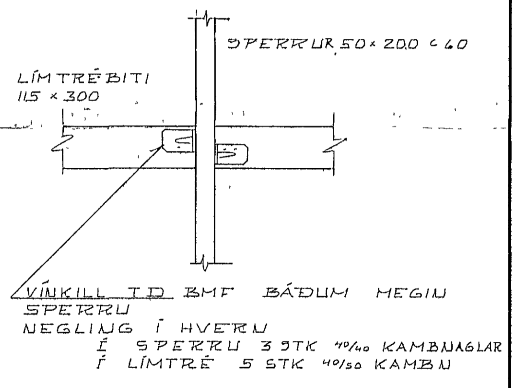
SÉRMYND II 1:10
