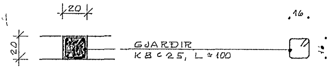
SÚLA S.1 1:20
