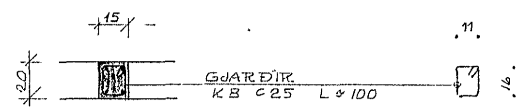
SÚLA S.2 1:20
