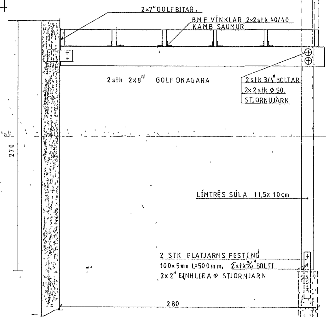
SNID A-A 1:20
