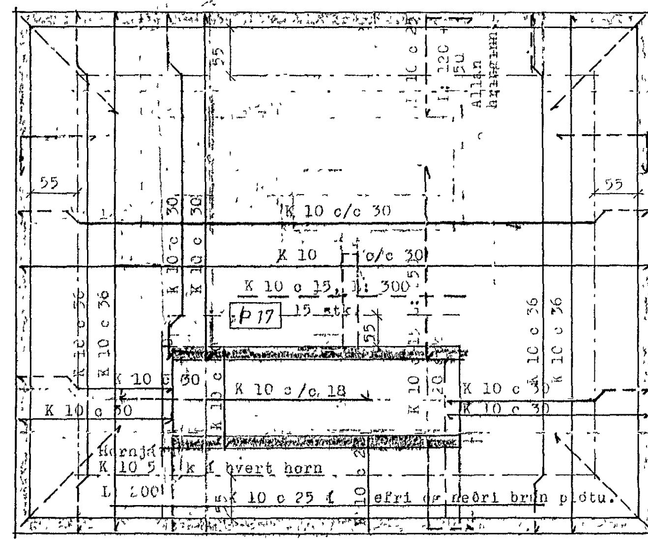
PLATA YFIR KJALLARA 1:50
