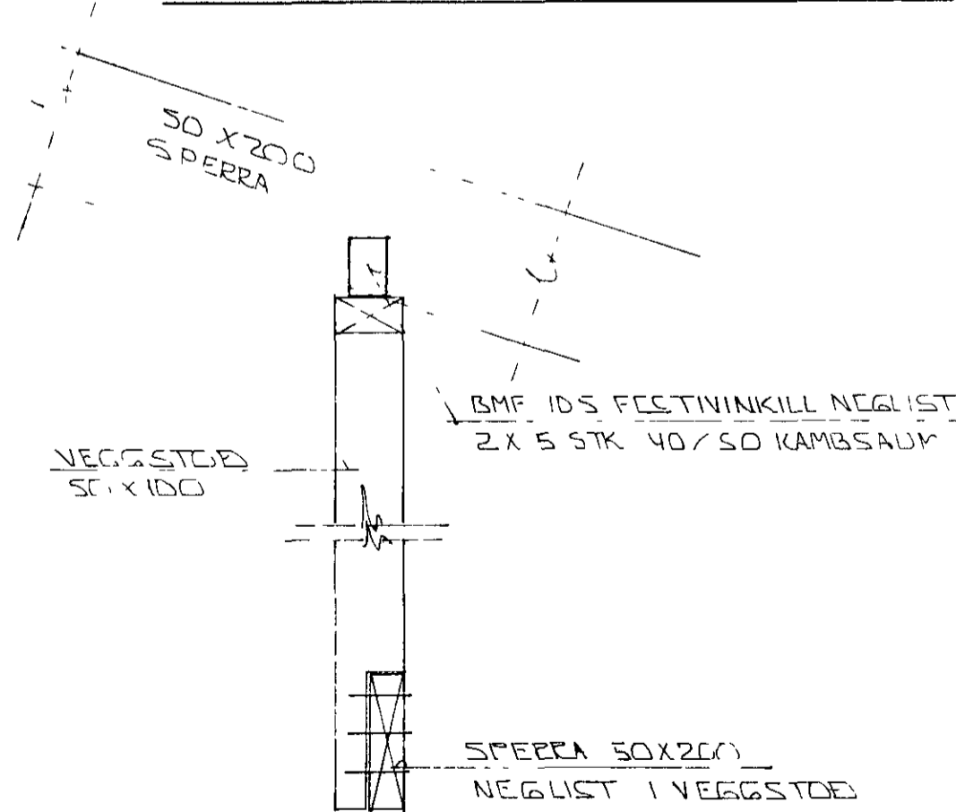
GRUNNMYND ÞAKVIRKIS 1:50
