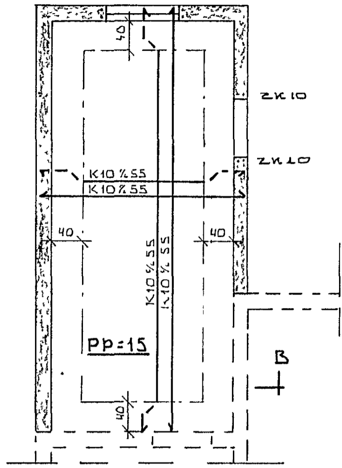
GRUNNMYND ~ 1:50 JARDHÆÐ
