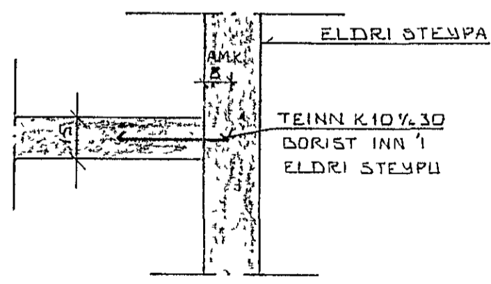
SNID B ~ 1:20
