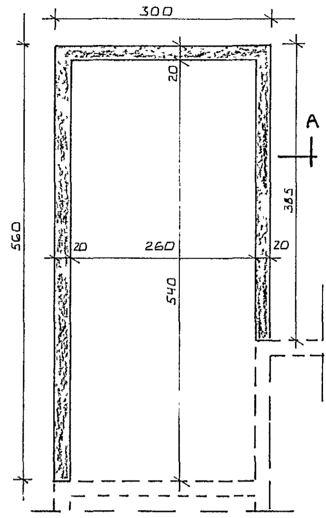
GRUNNMYND ~ 1:50 UNDIRSTÖÐUR
