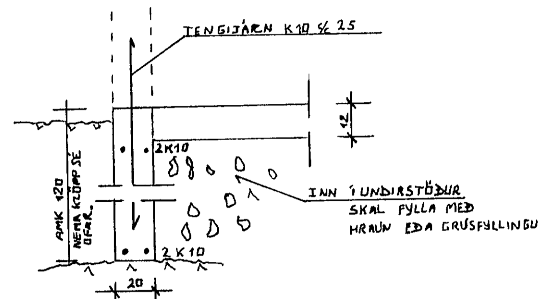
UNDIRSTÖÐUR 1:20
