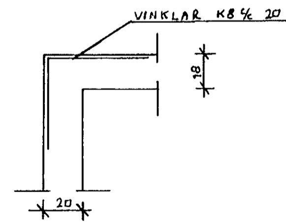
SNID B-B 1:20
